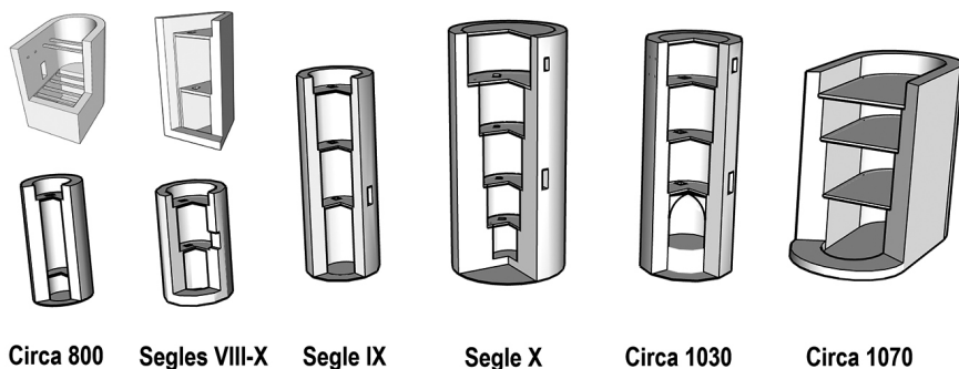
Figura 6. Proposta de seriació de les torres pallaresses. Font: autors.
