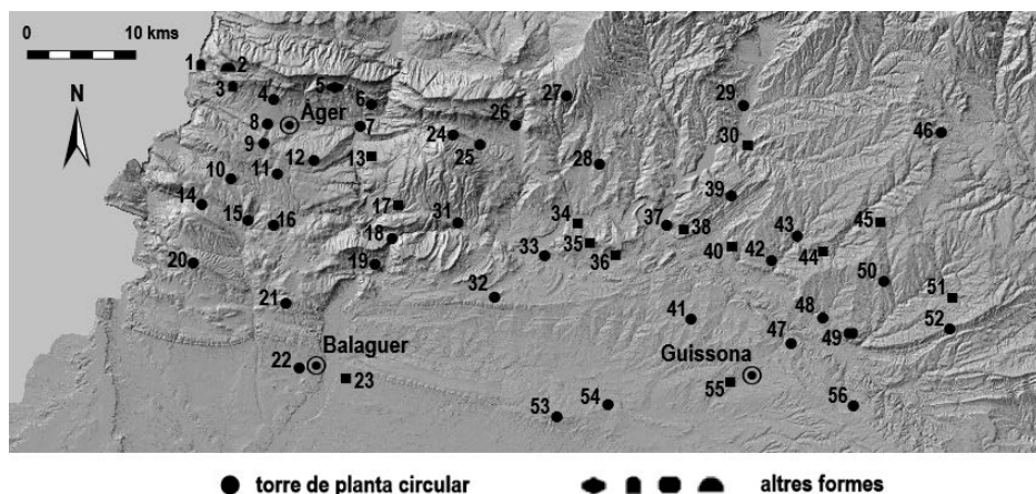
Figura 7. Fronts de la Noguera i el Solsonès: 1. Pertusa; 2. Sant Llorenç; 3. Claramunt; 4. Torre del Negre; 5. Mallabecs; 6. L'Escumó; 7. Sant Oïсме; 8. Torre Sanui; 9. Montlleó; 10. Masos de Millà; 11. Fontdepou; 12. Cas; 13. Fontllonga; 14. Alberola; 15. Tartareu; 16. Secardit; 17. La Maçana; 18. Mont-roig; 19. Sant Salvador; 20. Cérvoles; 21. Campvim; 22. Erals de Balaguer; 23. La Ràpita; 24. Örenga; 25. Castelló de Meià; 26. Meià; 27. Comiols; 28. Montmagastre; 29. Aguilar; 30. Ansamora; 31. Alòs; 32. Torre de n'Eroles; 33. Artesa; 34. Vilves; 35. Grialó; 36. Cargol; 37. Ponts; 38. Valldans; 39. Valldàries; 40. La Figuera; 41. Vilamajor; 42. Sanaüja; 43. Sallent; 44. Lloberola; 45. Peracamps; 46. Castellvell de Solsona; 47. Talteüll; 48. La Granja; 49. L'Aguda; 50. Vallferosa; 51. Ardèvol; 52. Castellanes; 53. Almenara; 54. Castellnou d'Ossó; 55. La Morana; 56. Ivorra. Font: autors.
