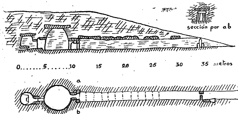
Cueva del Romeral. (Sección y planta.) Sepulcro en cúpula.
