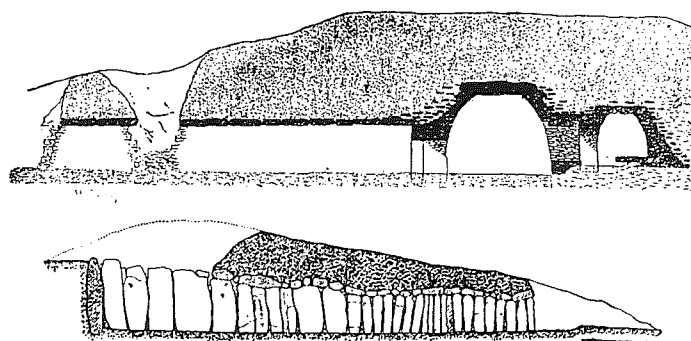
Evolución de los monumentos megalíticos. Arriba: sepulcro de cúpula del Romeral, en la comarca de Antequera; abajo: dolmen de Soto, en la comarca de Huelva. Las secciones muestran la diferencia de riqueza y técnica constructiva entre las sepulturas de falsa cúpula y los dólmenes.
