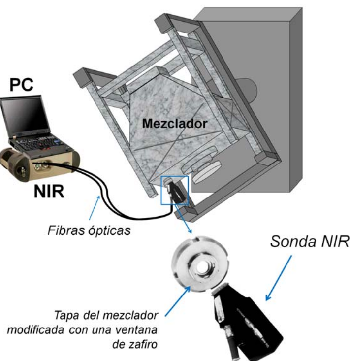
Figura 5.2. Esquema del modo de registro de los espectros NIR en el mezclador industrial.
