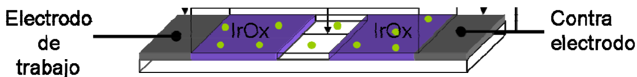
Figura 2.12 Esquema de la configuración usada para la electroestimulación de neuronas corticales sembradas sobre capas de IrO x
