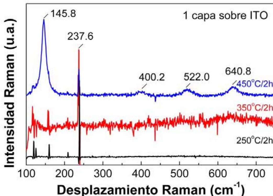
Figura 3.10 Espectro Raman de capas de \text{TiO}_2 sobre ITO tratadas a diferentes temperaturas.
