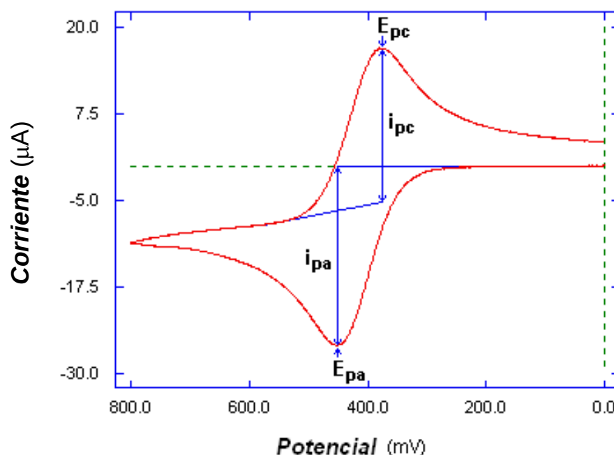
Figura 2.4 Esquema general de una voltametría cíclica.
