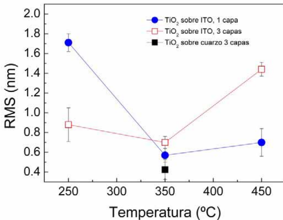
Figura 3.14 Curva del factor de rugosidad RMS con respecto a la temperatura de tratamiento para capas de \text{TiO}_2 sobre ITO y cuarzo.
