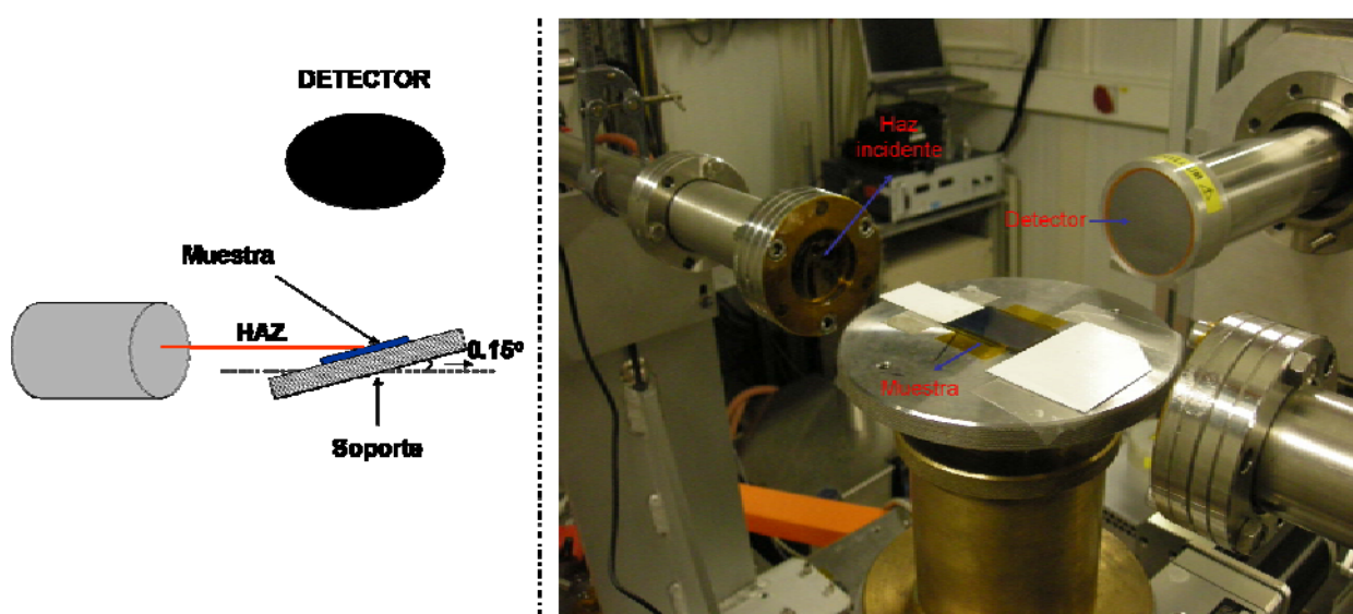
Figura 2.9 Configuración utilizada en las medidas de XAS de muestras de \text{IrO}_x .
