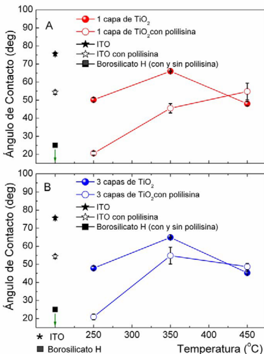
Figura 3.18 Curvas del ángulo de contacto con medio de cultivo en capas de \text{TiO}_2 sobre ITO con y sin polilisina A) 1 capa y B) 3 capas
