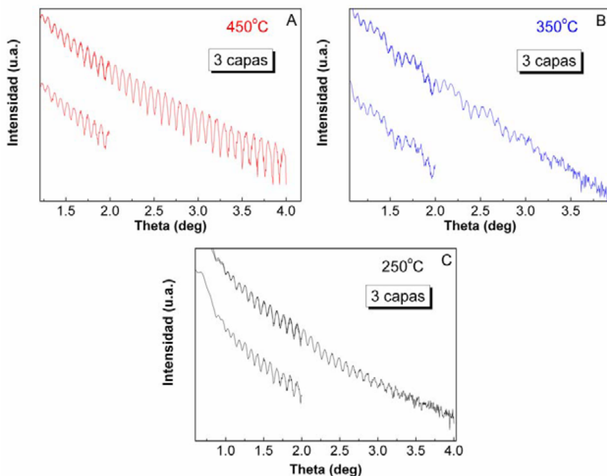
Figura 3.4 Curvas de reflectometría de rayos X de capas de \text{TiO}_2 tratadas a A) 250°C, B) 350°C y C) 450°C.
