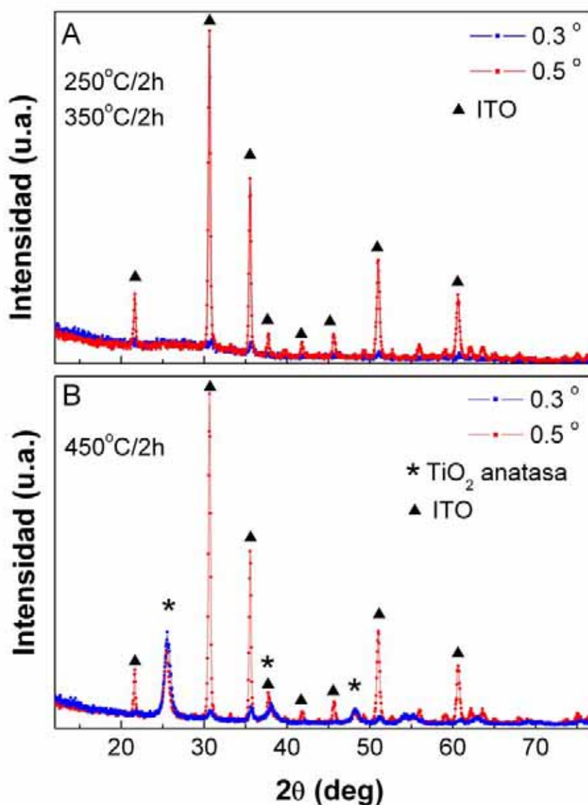
Figura 3.5 Difractogramas de Rayos X de ángulo rasante de capas de \text{TiO}_2 tratadas a A) 250^\circ\text{C} y 350^\circ\text{C} durante 2 horas y B) 450^\circ\text{C} durante 2 horas.
