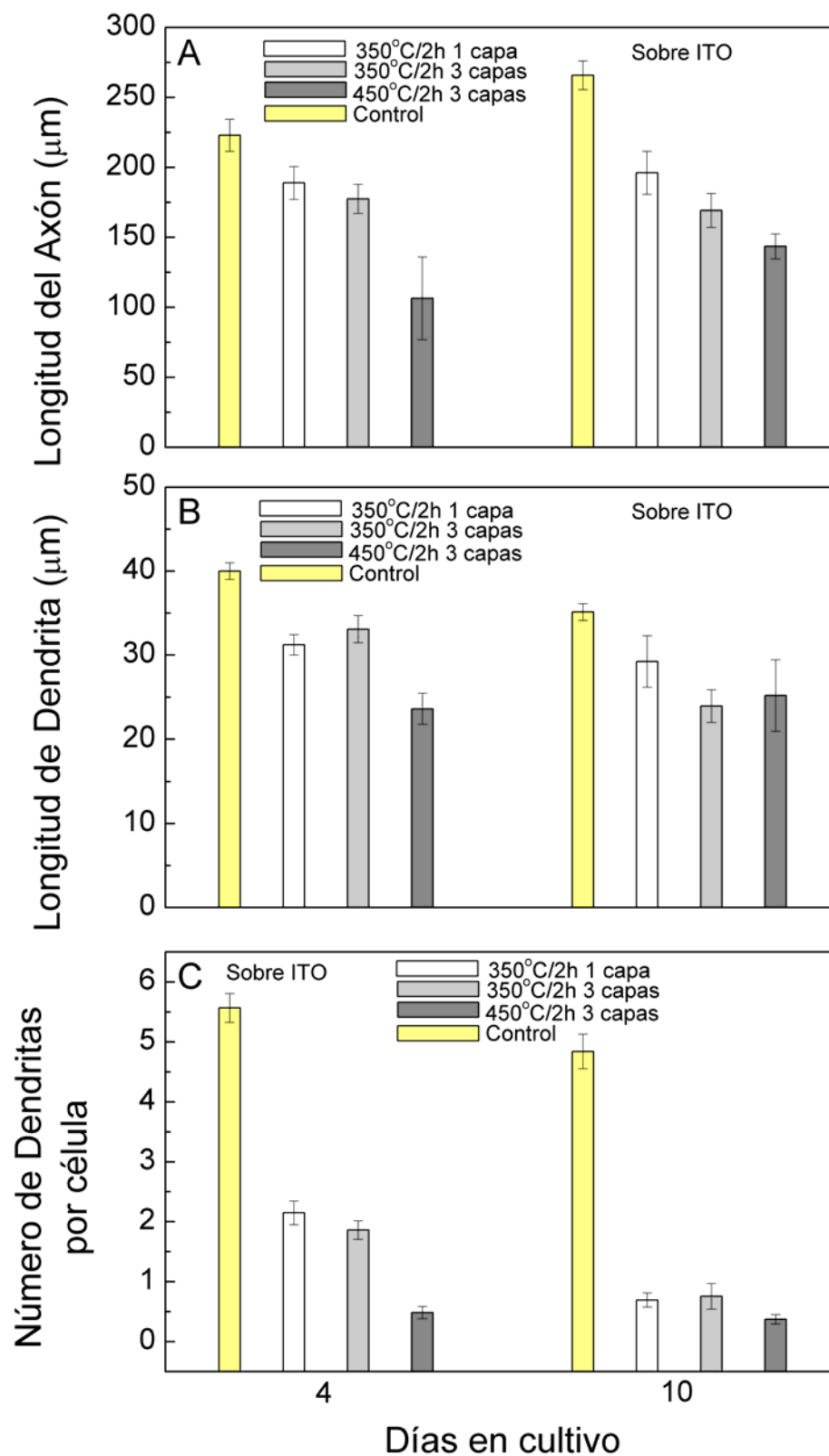
Figura 3.22 Procesos de crecimiento neuronal en cultivos de baja densidad ( 500 \text{ cel}/\text{cm}^2 ) en capas de \text{TiO}_2 y superficies de control. Los datos representan la diferencia media \pm desviación estándar del error significativa a p < 0.05 de: A) Longitud del axón primario, B) Longitud de las dendritas primarias y C) Número de dendritas primarias por célula.
