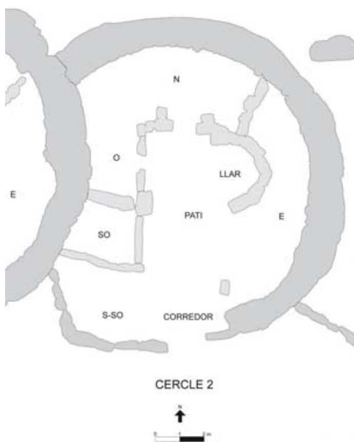
Plànol del Cercle 2 de Sant Vicenç d'Alcàidús (segons Plantalamor, 1991)
