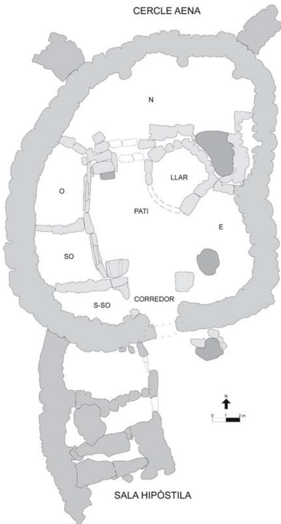
Plànol de la Casa AENA de Biniparratx Petit (segons de Nicolàs, 1995)
