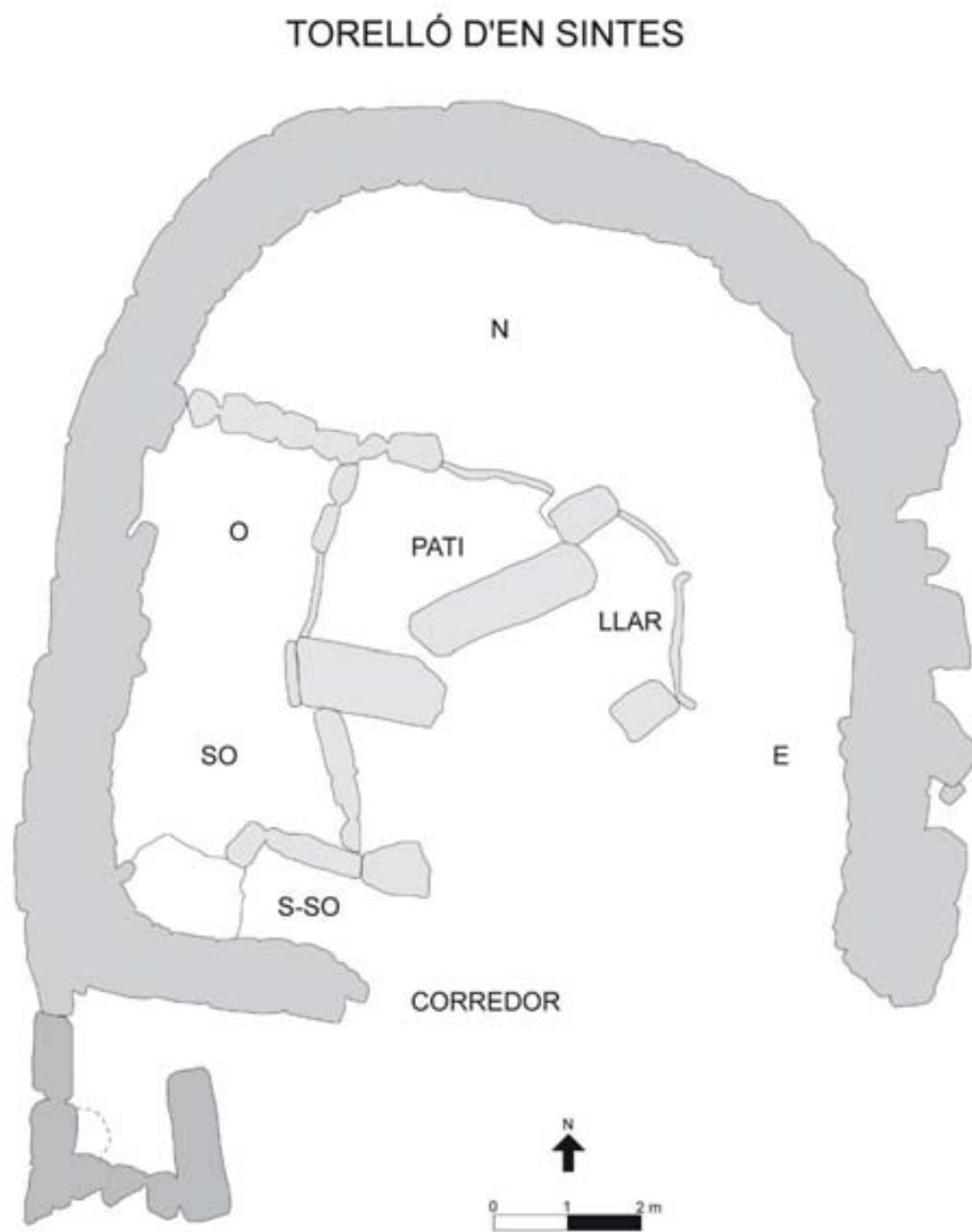
Plànol de la casa de Torelló d'en Sintes (segons Plantalamor, 1991)
