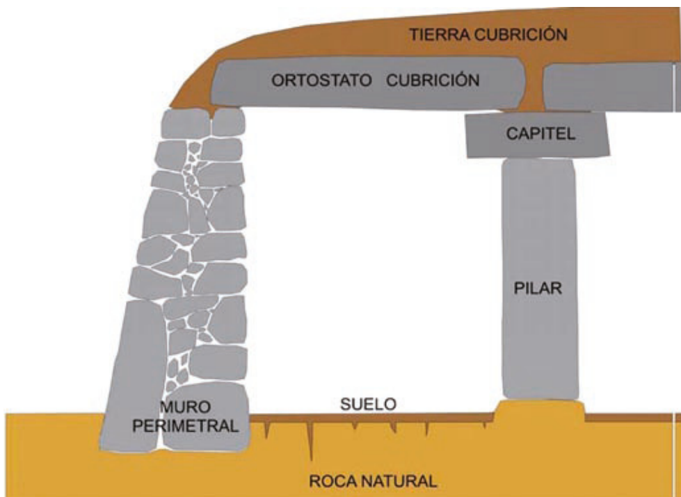
Esquema de com es cobriria l'Edifici 2 (Pérez-Juez, 2011)
