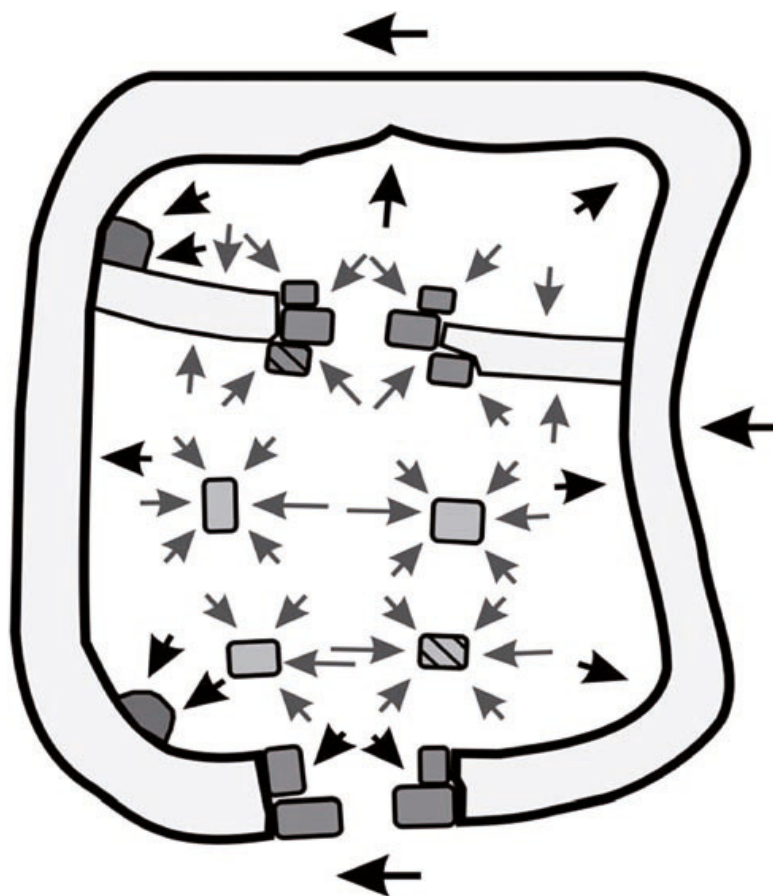
Esquema del repartiment de forces proposat per l'equip de Boston University per tal de suportar la coberta de l'Edifici 2 (Pérez-Juez, 2011)
