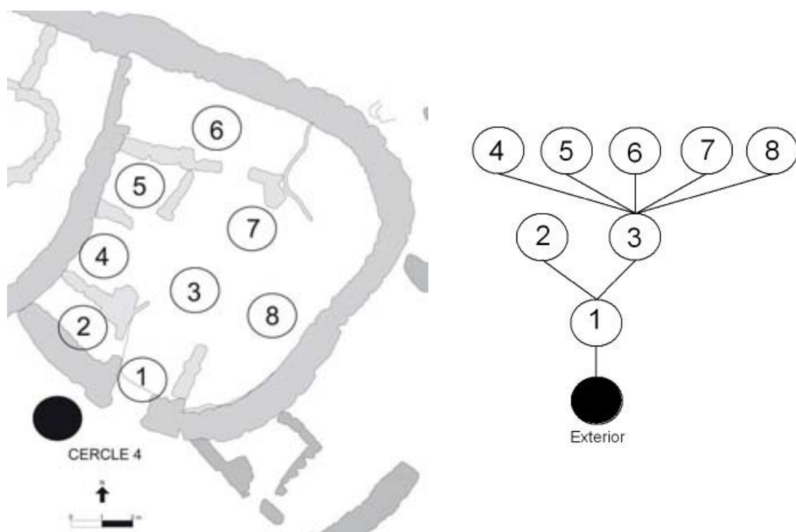
Esquema de circulació del Cercle 4 de Sant Vicenç d'Alcaldús
