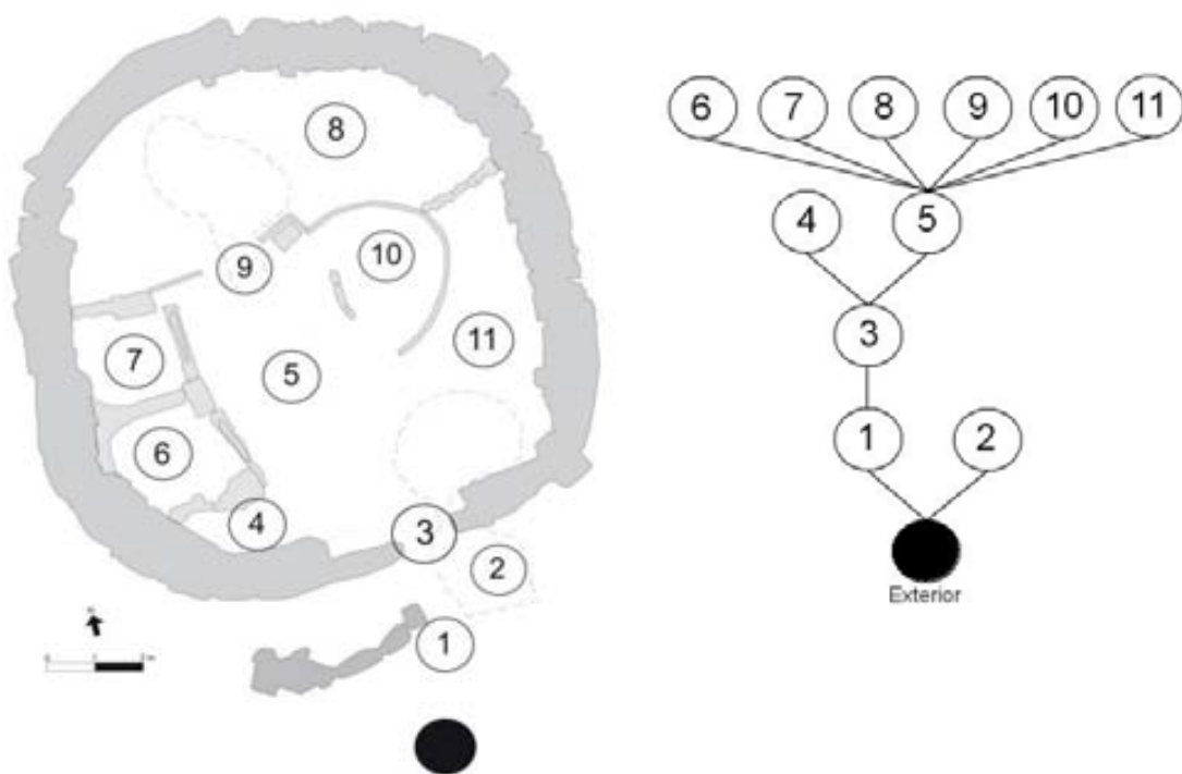
Esquema de circulació de la Casa Serra Belabre de Biniparratx Petit
