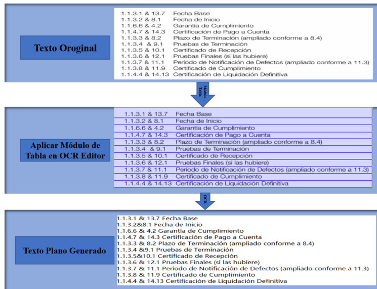
Figura 7.8: Ejemplo de aplicar la plantilla de tabla. (Elaboración propia)
