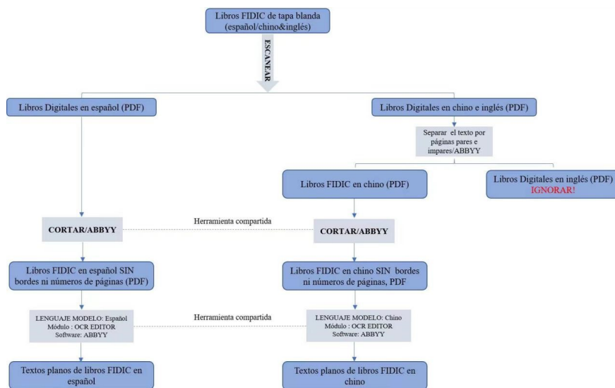
Figura 7.1: Pasos para Convertir los Documentos de PDF a Texto Plano. (Elaboración propia)
