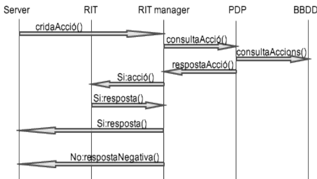
Fig3. Diagrama de seqüència del procés per a executar el codi del client.
