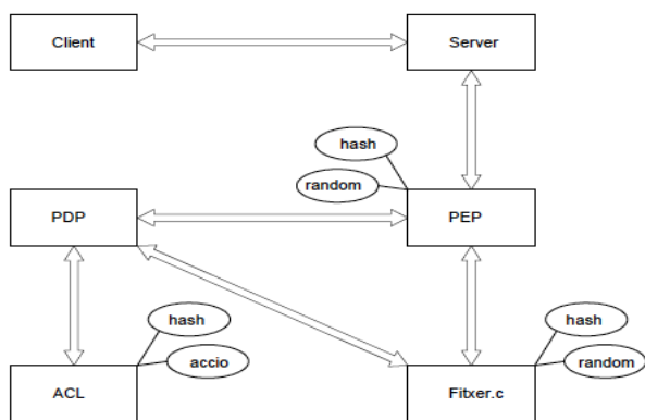
Fig6. Esquema del mòduls i les seves comunicacions per la tercera part de la implementació.
