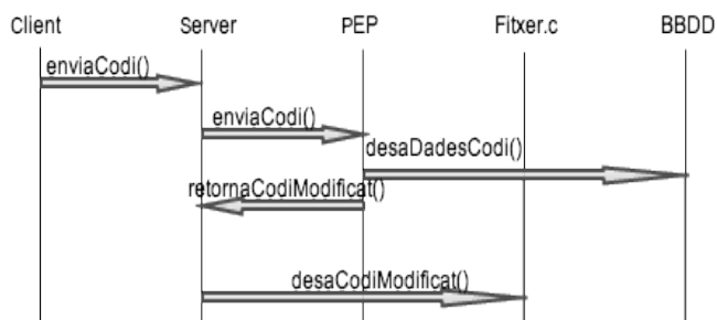
Fig2. Diagrama de seqüència del procés per desar el codi que posteriorment s'executarà.
