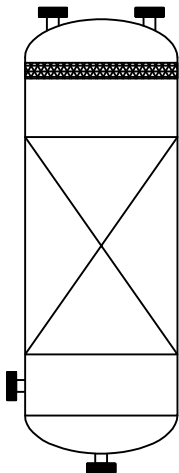
TORRE D'ABSORCIÓ
