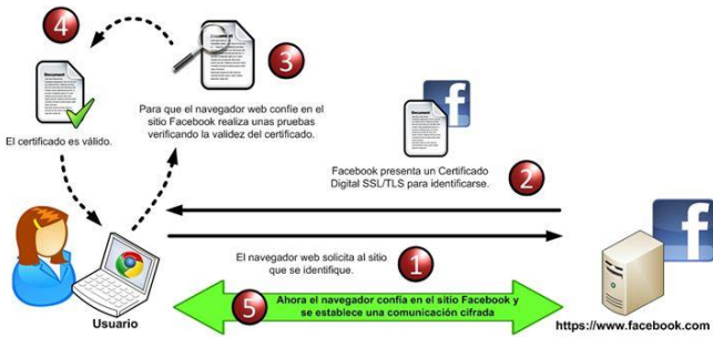
Fig. 2. Proceso básico enumerado para iniciar una conversación cifrada cliente-servidor, utilizado en el acceso a Facebook [14]
