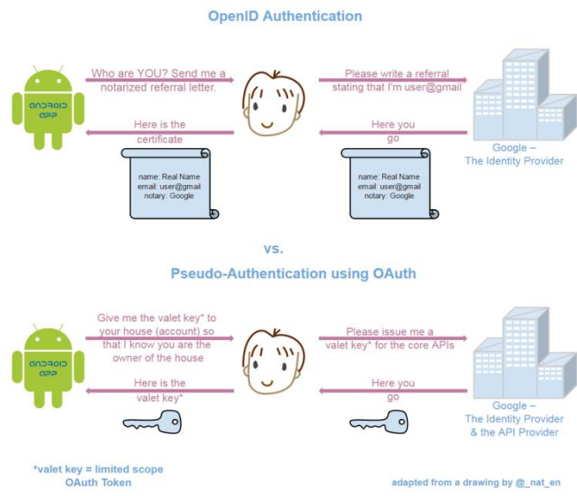
Fig. 1. Comparación entre la autenticación de OpenID y la pseudoautenticación de OAuth.
