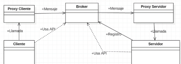
Figura 3. Diagrama patrón de diseño bróker
