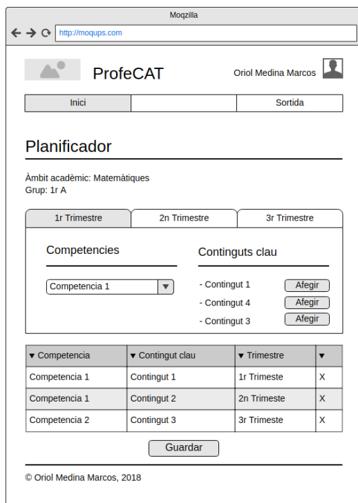
Fig. 3: Mockup de la pantalla "Planificador"
