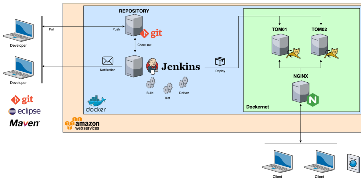
Fig. 3. Arquitectura del sistema
