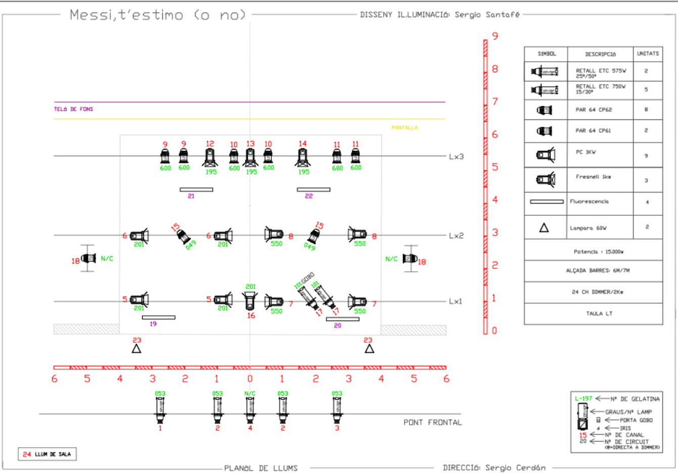
Imagen 20: Plano de luces obra de teatro "Messi t'estimo (o no)" Autor: Sergio Santafé
