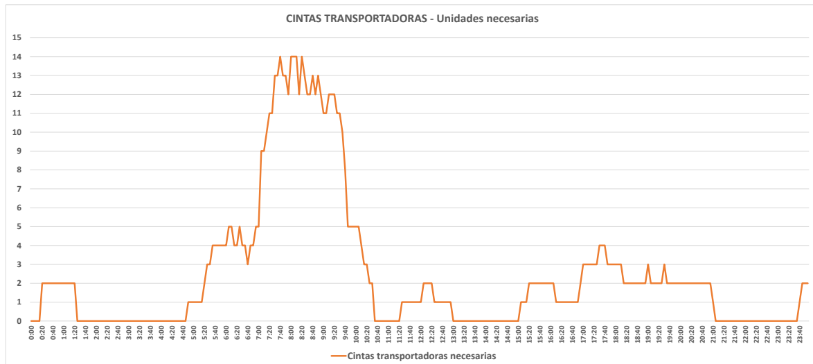
Figura 51. Cintas transportadoras. Unidades necesarias por franja horaria.
