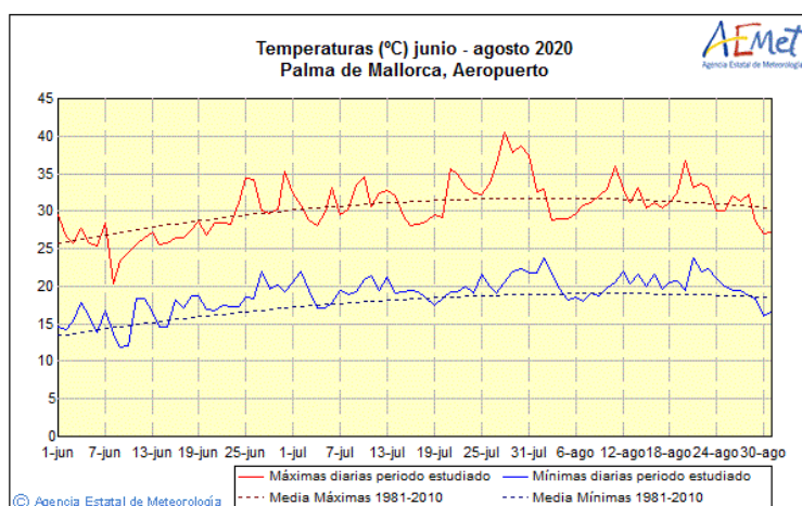
Figura 47. Temperatura Aeropuerto Palma. Junio – Agosto 2020 11
