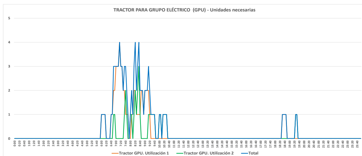
Figura 60. Tractores para grupos eléctricos (GPU). Unidades necesarias por franja horaria.
