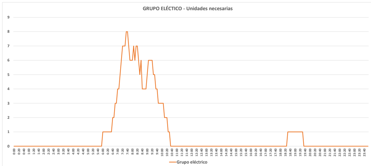
Figura 59. Grupos eléctricos (GPU). Unidades necesarias por franja horaria.
