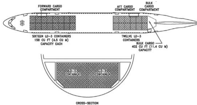
Figura 45. Boeing 788 y Boeing 789. ULDs a utilizar 10
