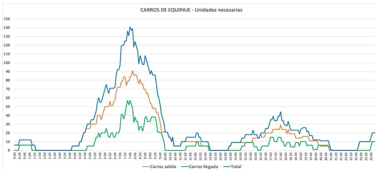
Figura 53. Carros de equipaje. Unidades necesarias por franja horaria.
