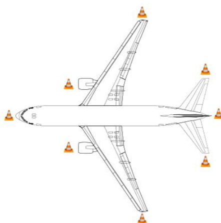
Figura 50. Disposición de conos en la aeronave
