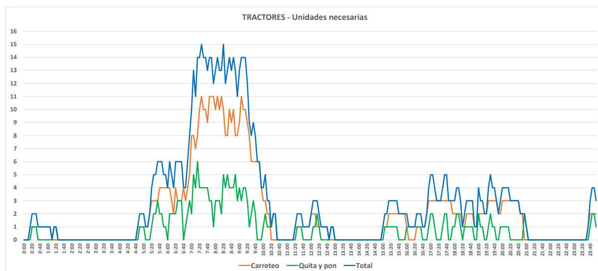
Figura 52. Tractores. Unidades necesarias por franja horaria.
