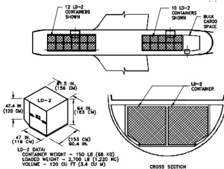
Figura 44. Boeing 763. ULDs a utilizar 9
