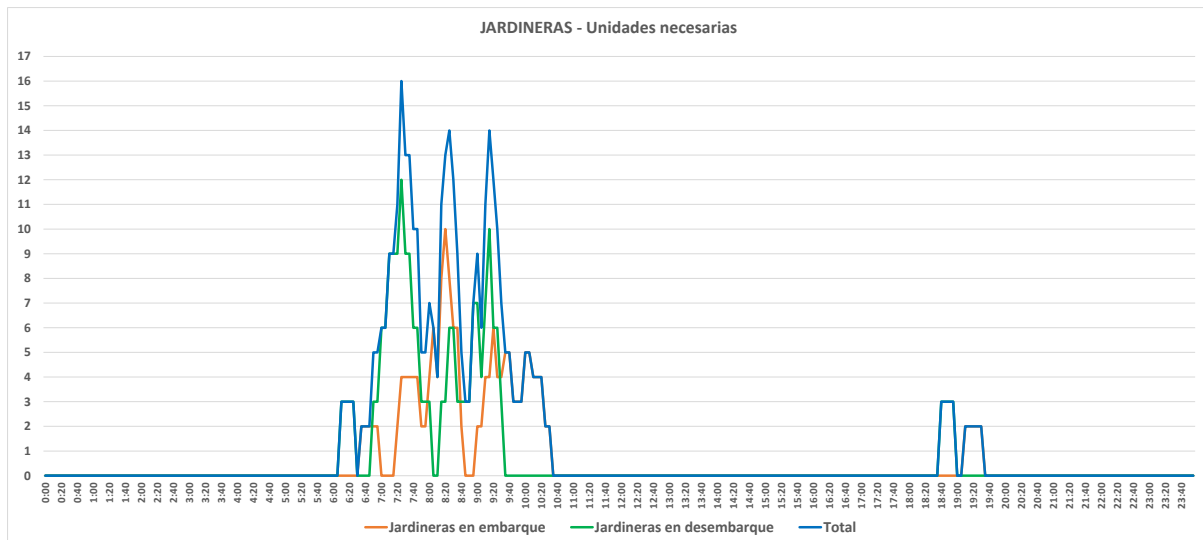
Figura 57. Jardineras. Unidades necesarias por franja horaria.
