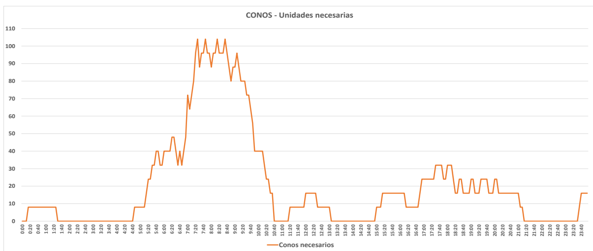
Figura 55. Conos. Unidades necesarias por franja horaria.
