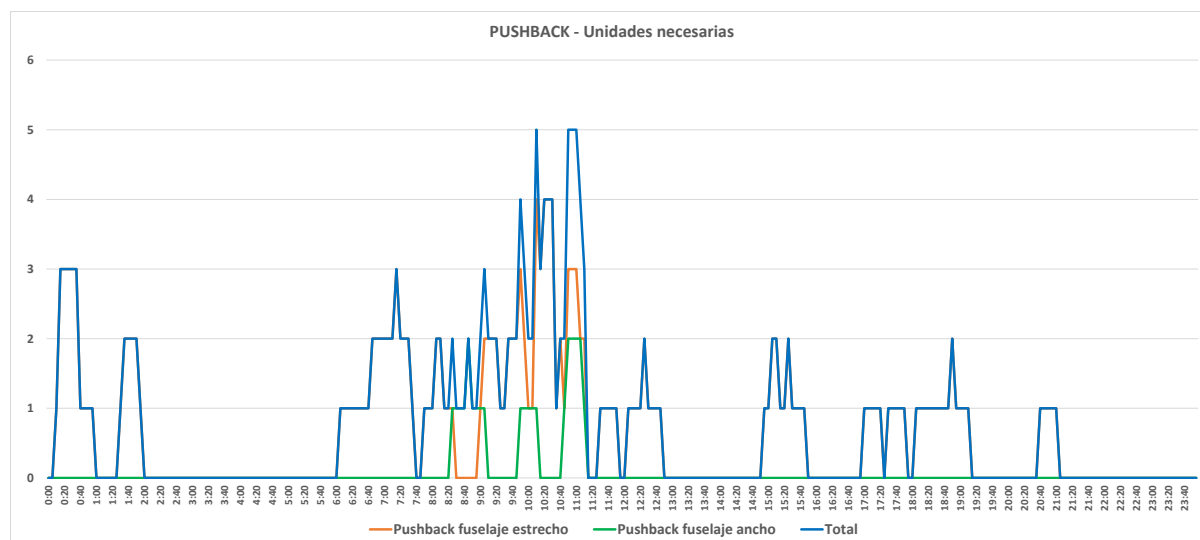
Figura 61. Pushback. Unidades necesarias por franja horaria.
