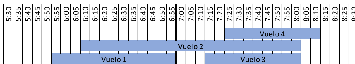
Figura 16. Evolución temporal de las escalas del 02/01/2022
