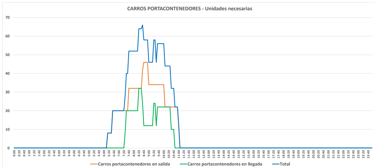
Figura 65. Carros de equipaje. Unidades necesarias por franja horaria.
