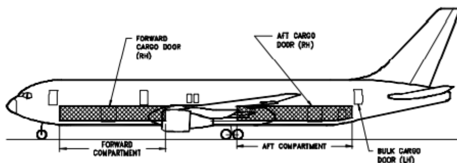
Figura 43. Boeing 763. Situación bodegas de carga 8
