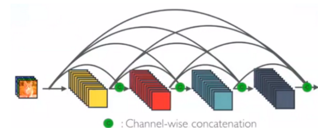
Fig. 1: Estructura d'una connexió densa (font: https://towardsdatascience.com/review-densenet-image-classification-b6631a8ef803 )
