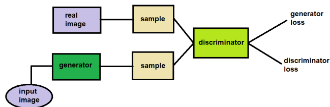
Fig. 2: Estructura d'una GAN
