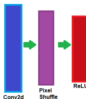
Fig. 7: Estructura de l'últim block del Generador
