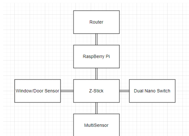
Imagen 5: Conexiones Hardware.
