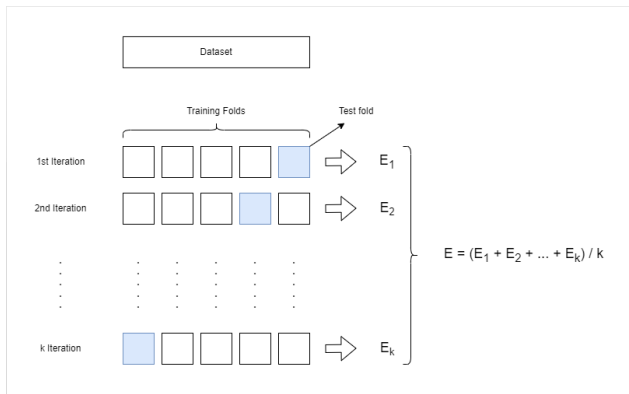
Fig. 2: Mètode K-Fold Cross Validation
