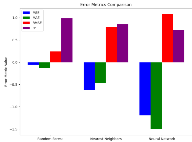
Fig. 3: Resultats K-Fold Cross Validation
