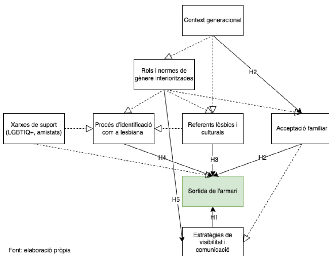
Figura 1: Model d'anàlisi
