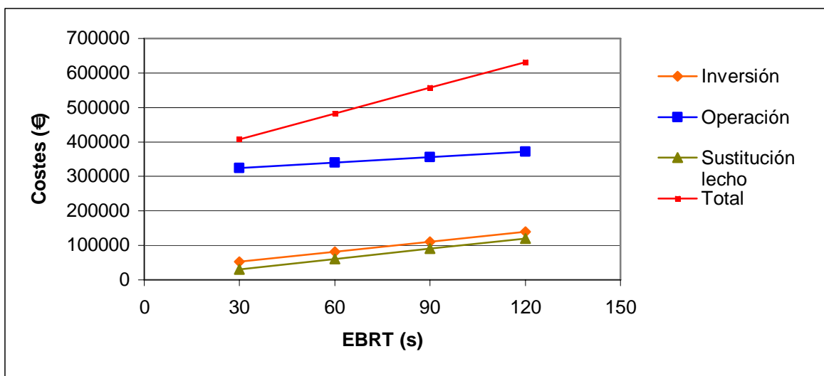
Figura 4.7 Costes básicos en función del tiempo de residencia (EBRT)
