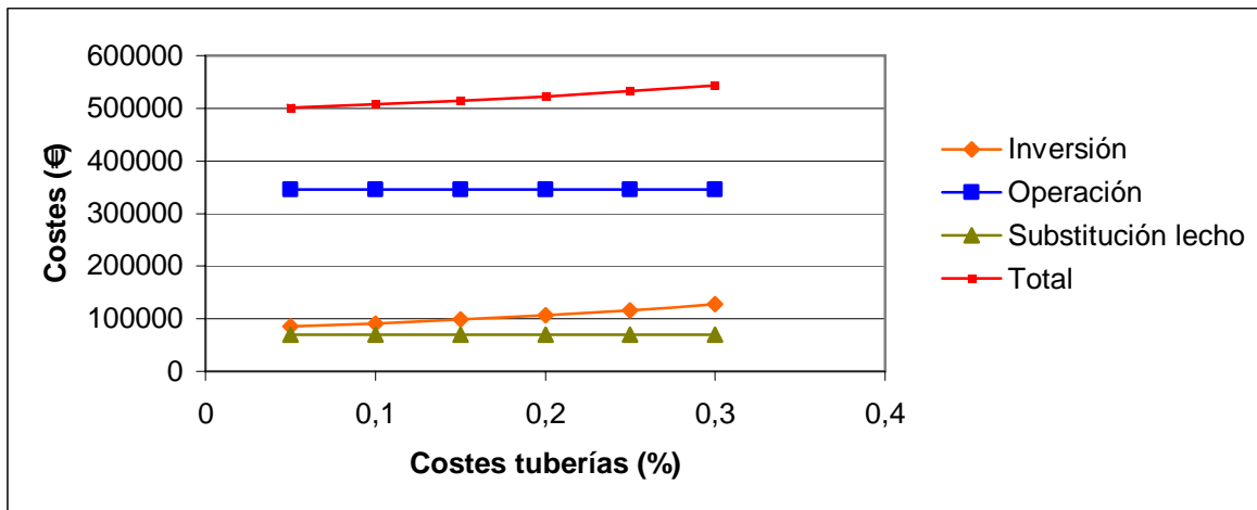
Figura 4.20 Costes principales variando el % de costes de las tuberías respecto de los costes totales de inversión.
