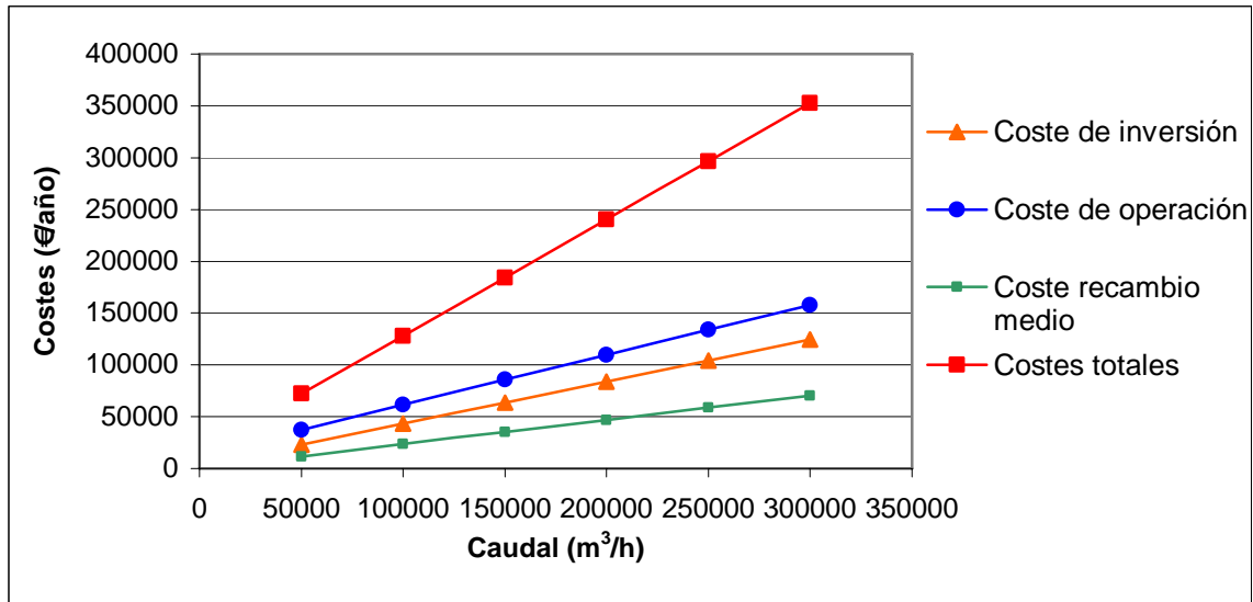
Figura 4.3 Representación gráfica de los costes principales variando el caudal de diseño del biodepurador de gases.
