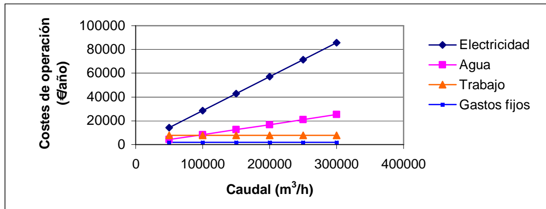
Figura 4.4 Diagrama del porcentaje de los costes implicados en el coste anual de operación a diferentes caudales.
