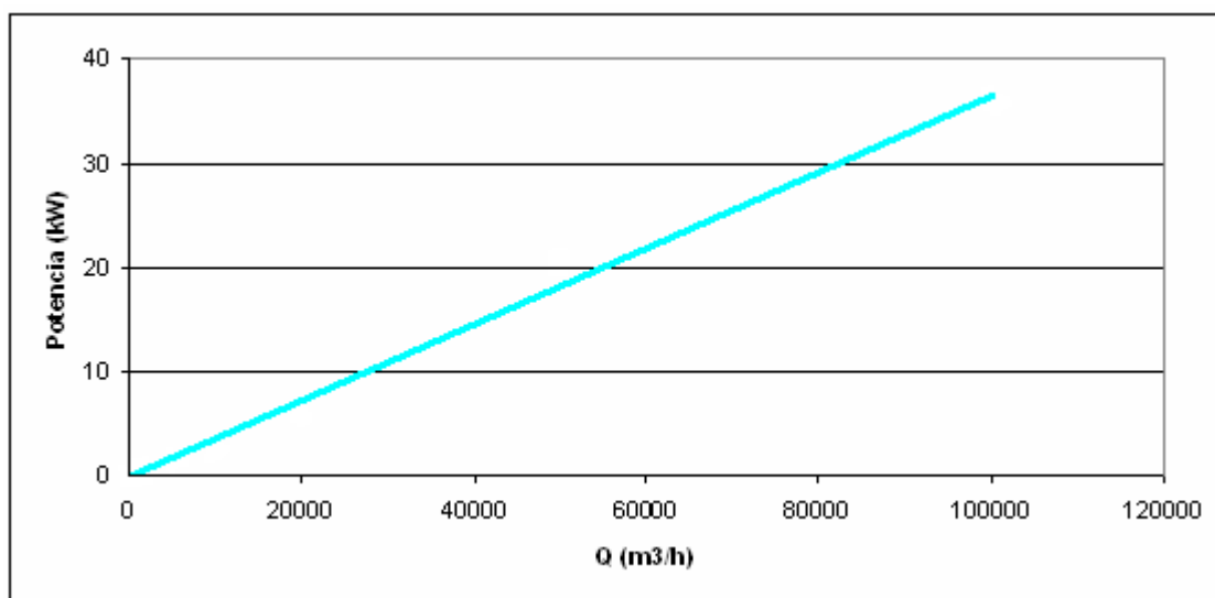
Figura 3.3 Consumo de una soplante en función del caudal de gas a tratar. En el anexo A se explica cómo se ha obtenido este diagrama
