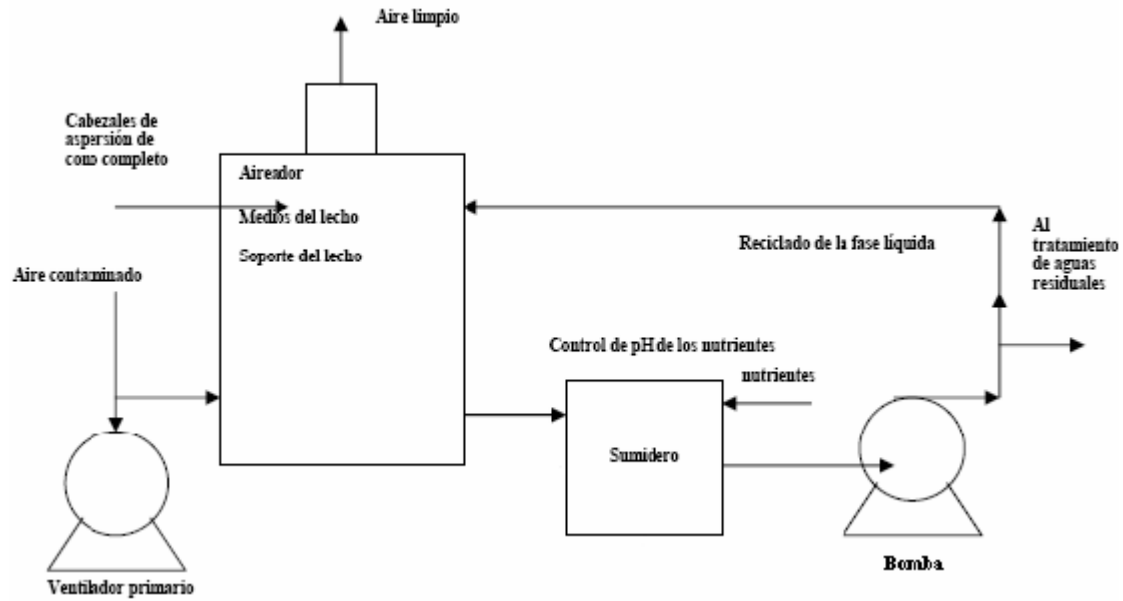
Figura 1.9 Sinopsis del tratamiento de gases aerobio de un biodepurador (www.epa.gov)
