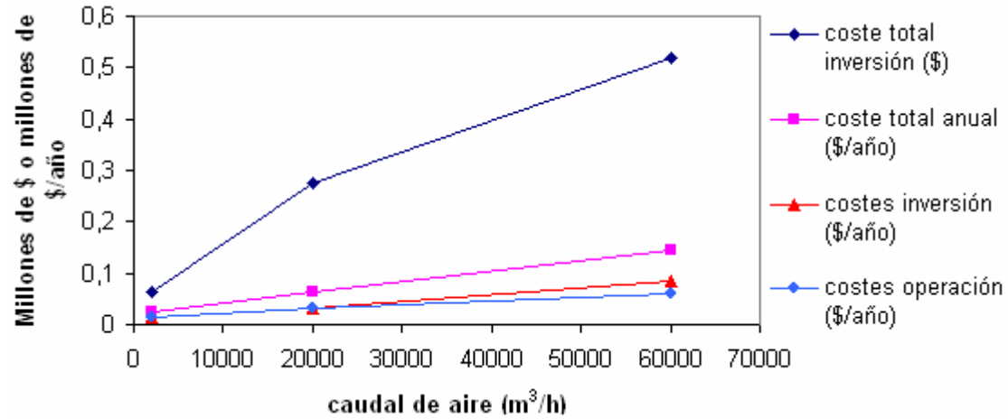
Figura 1.11 Costes anuales totales en función del caudal de entrada de gas que contiene contaminantes fácilmente biodegradables (Devanny, 1999).
