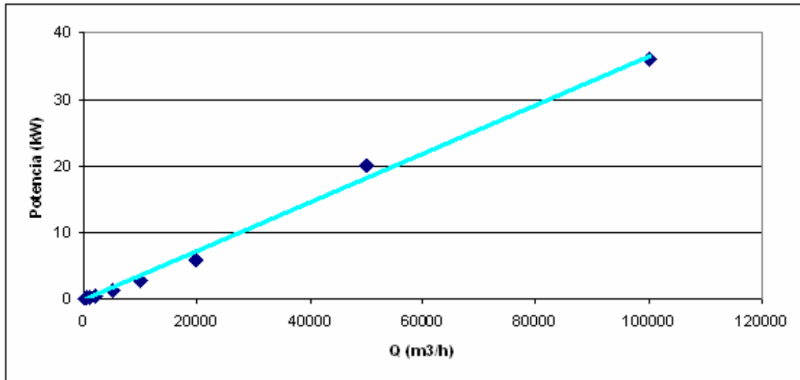
Figura 7.3 Representación de unos cuantos puntos del diagrama caudal vs. Potencia de la figura anterior y su recta de regresión lineal. El objeto de esta gráfica es minimizar el error visual del individuo a buscar visualmente los valores de la potencia en función de su caudal.
