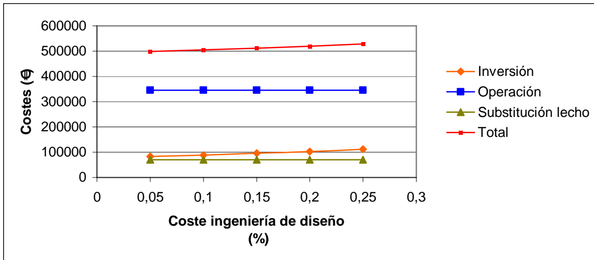
Figura 4.23 Costes básicos en función del % de los costes de ingeniería de diseño.
