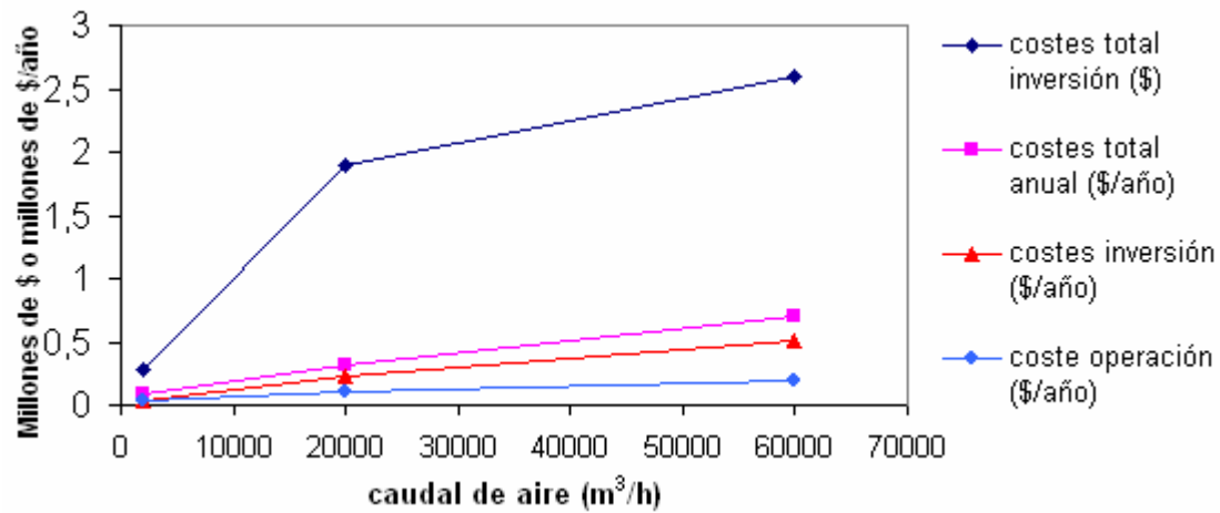
Figura 1.12 Costes anuales totales en función del caudal de entrada de gas que contiene contaminantes difícilmente biodegradables (Devanny, 1999).
