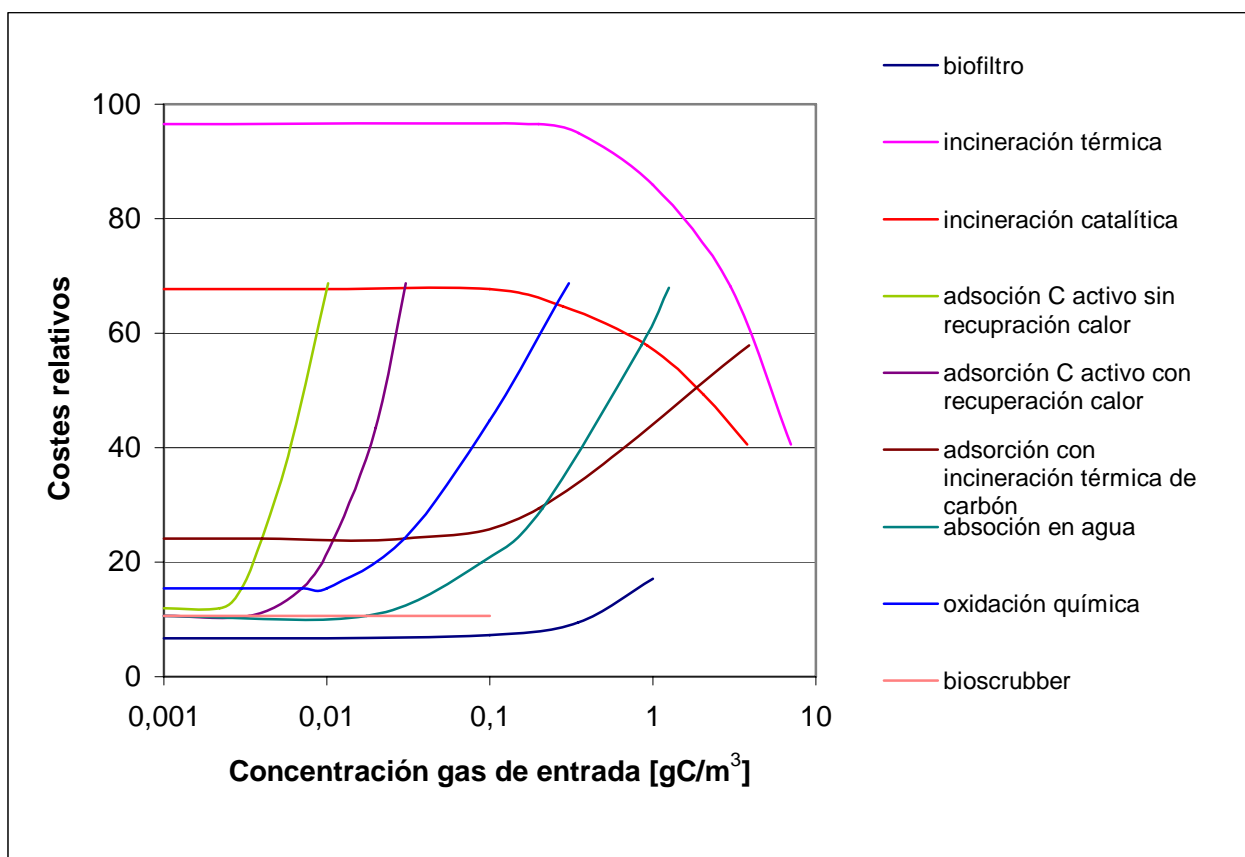
Figura 1.10 Comparación de los costes relativos de diversas técnicas de purificación de gas residual. Caudal de gas 40,000 \text{m}^3/\text{h} , nivel de precio 1982 (Deshusses, 1994).
