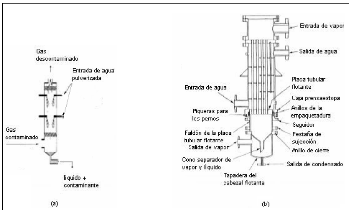
Figura 1.3 Equipos de condensación para depuración de gases. a) Condensador de contacto. Tal como se representa en el diagrama el gas entra en contacto con el líquido refrigerante condensando así la parte contaminante del gas. El condensado y el líquido bajan a la parte inferior y por arriba sale el gas limpio; b) Condensador de superficie. Gas contaminante y líquido refrigerante entran desde arriba. El líquido circula a través de tuberías en la superficie de las cuales condensa el contaminante cayendo con el líquido por la parte de abajo. El gas limpio escapa por la parte de abajo (Font, X. Curso 2005-2006. Tècniques de Tractament i Depuració d'Emissions.UAB).
