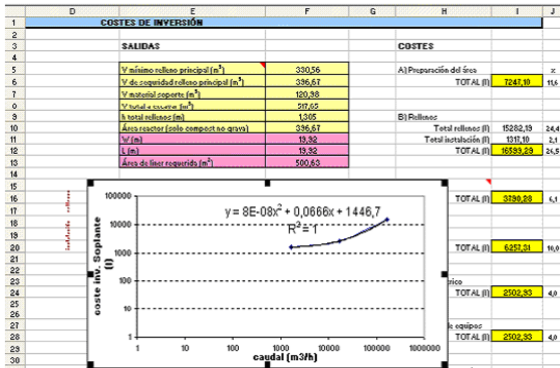
Figura 3.3 Entorno de trabajo en el que nos movemos para realizar los costes de construcción y operación a partir de parámetros de diseño. Concretamente esta hoja de cálculo corresponde a los costes de inversión como se puede observar.
