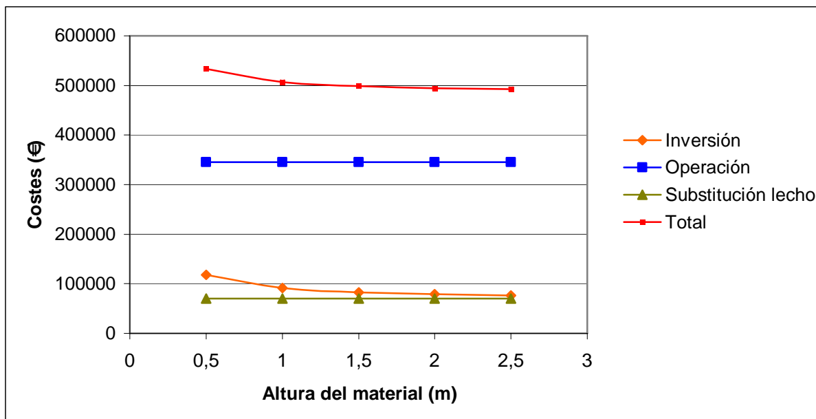
Figura 4.13 Costes principales variando la altura del relleno.
