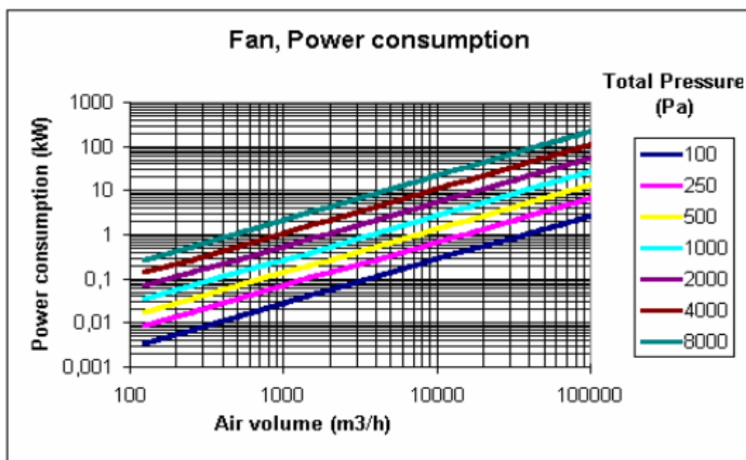
Figura 7.2 Diagrama en el que se muestra la potencia de una soplante en función de su caudal para diferentes presiones totales. En nuestro caso escogeremos la línea azul celeste ( http://www.engineeringtoolbox.com ).
