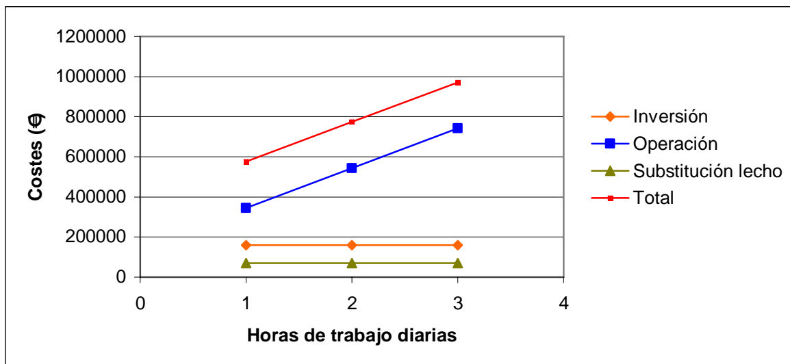
Figura 4.28 Costes principales dependiendo del tiempo horario dedicado a la manipulación del biofiltro.
