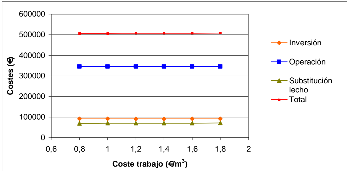
Figura 4.16 Costes totales variando los costes de trabajo.
