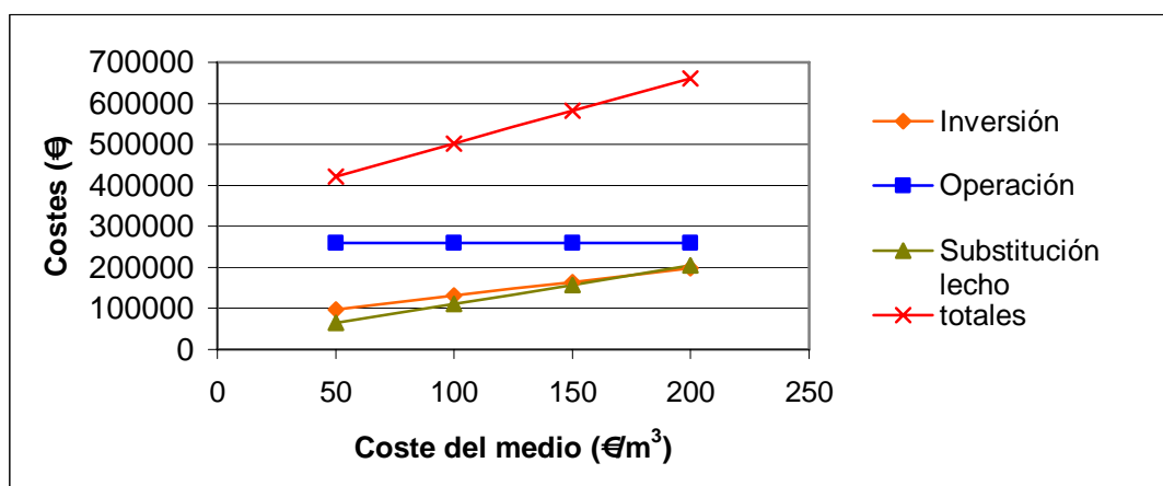
Figura 4.8 Variación de los costes principales aumentando el precio del medio
