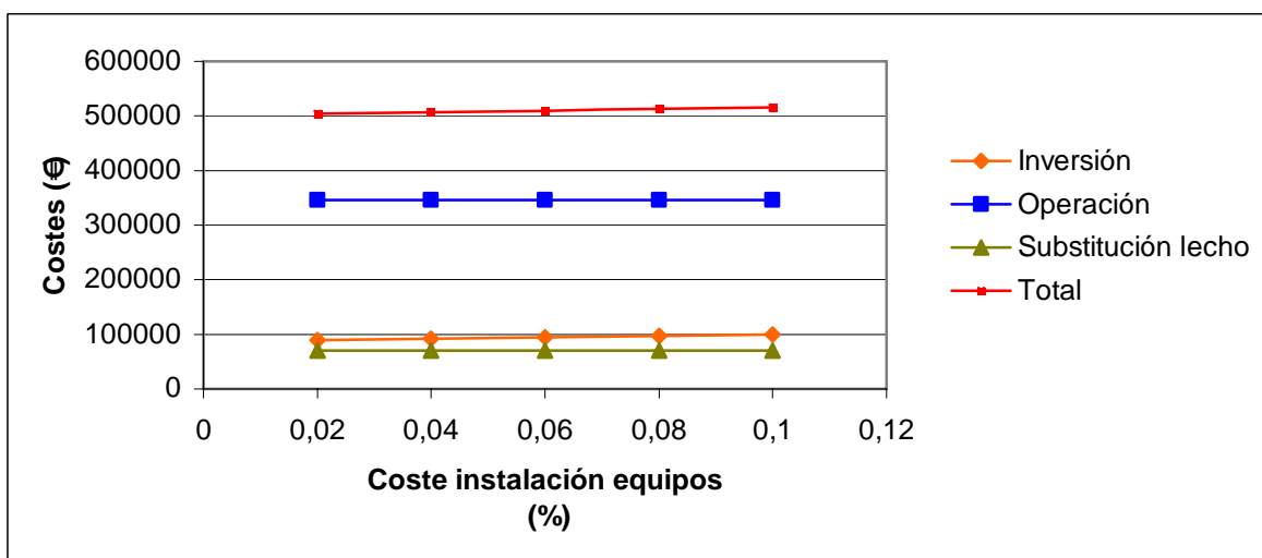
Figura 4.22 Costes fundamentales en función del porcentaje del coste de instalación de equipos referidos al coste de inversión total.
