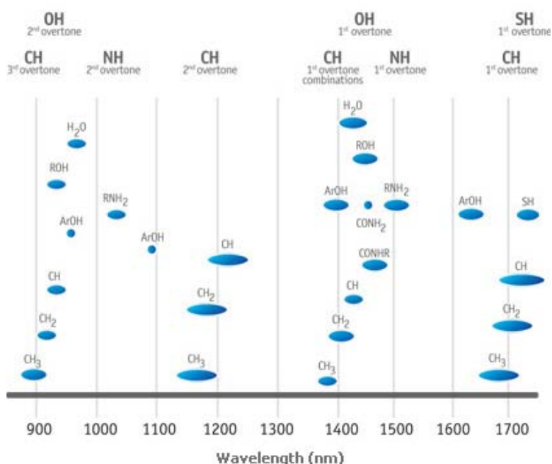
Figura 1.2. Bandes d'absorció al rang NIR d'estudi (900-1700 nm) 17 .
