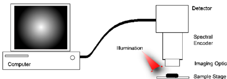
Figura 2.1. Esquema del muntatge de mesura 20 .
