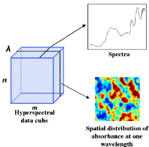
Figura 1.3. Esquema de la composició del hyperspectral cube 21 .
