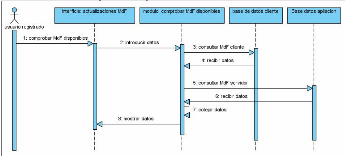
Fig. 3.8: Comprobar modelos de funcionamiento disponibles.
