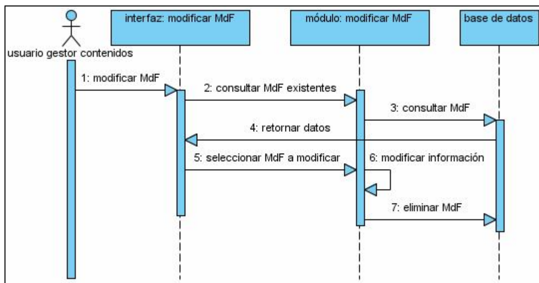
Fig. 3.18: Modificar modelos de funcionamiento.
