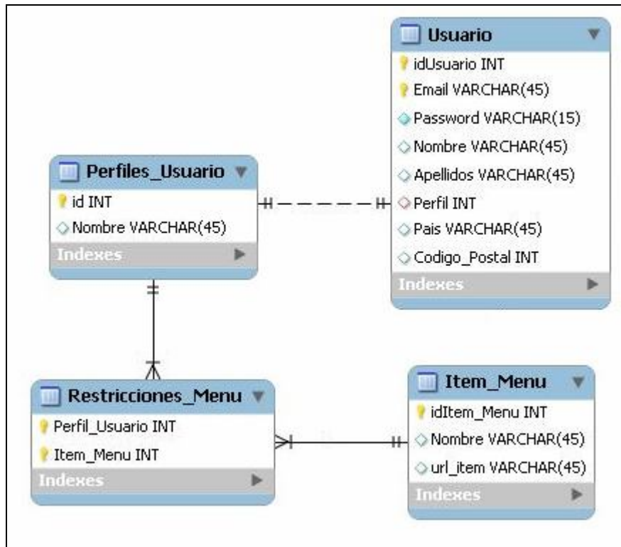
Fig. 5.8: Tablas para mostrar menú.
