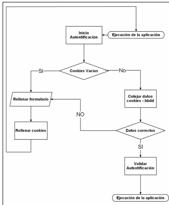
Fig. 5.2: Diagrama de flujo autenticación.
