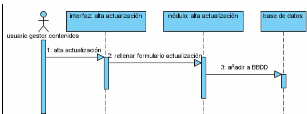
Fig. 3.19: Alta de actualización.
