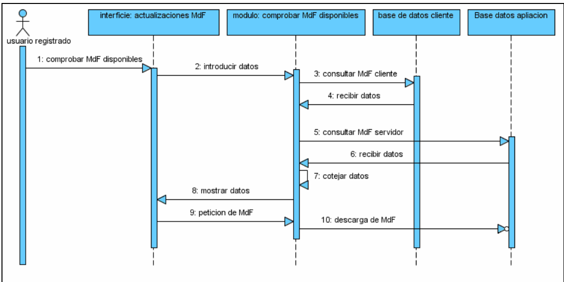
Fig. 3.9: Actualizar modelos de funcionamiento.
