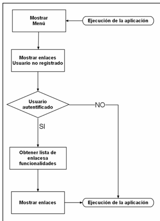
Fig. 5.4: Diagrama de flujo mostrar menú.
