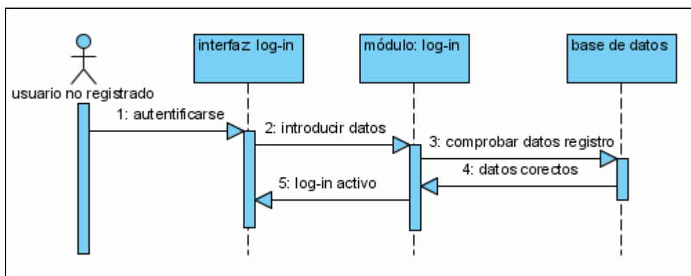
Fig. 3.4: Autenticarse
