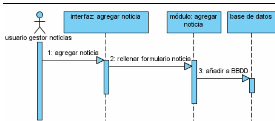
Fig. 3.10: Agregar noticia.
