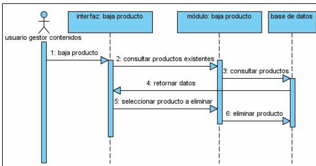
Fig. 3.14: Baja producto.
