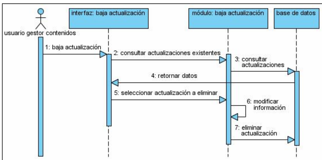
Fig. 3.21: Modificar actualización.
