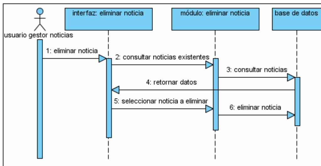
Fig. 3.12: Eliminar noticia.
