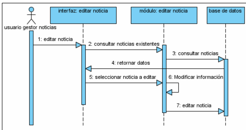
Fig. 3.11: Editar noticia.
