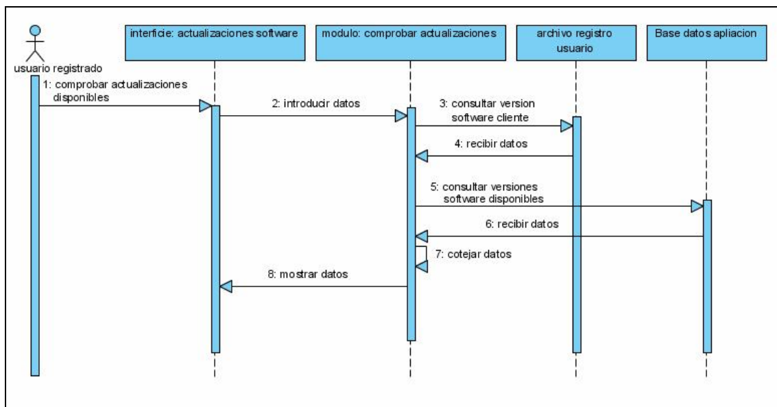
Fig. 3.6: Comprobar versiones de software.
