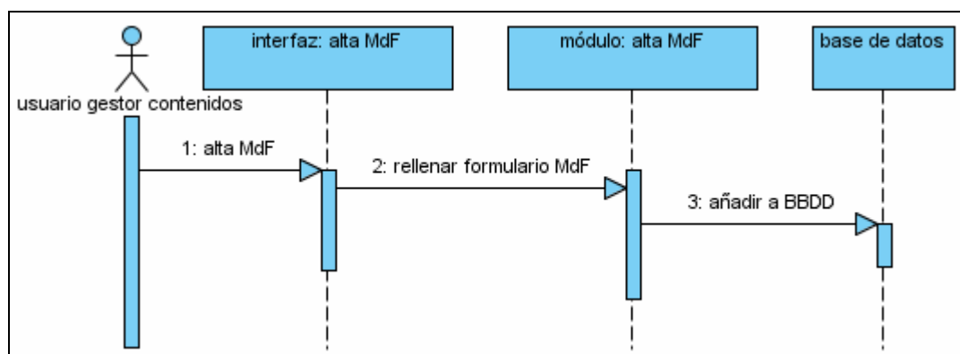
Fig. 3.16: Alta modelos de funcionamiento.
