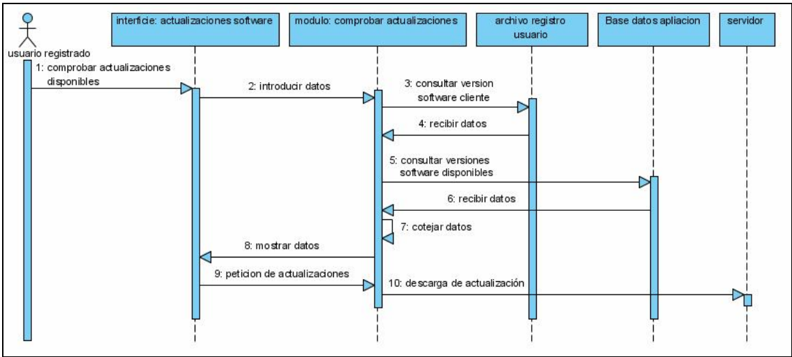
Fig. 3.7: Descargar actualizaciones de software.
