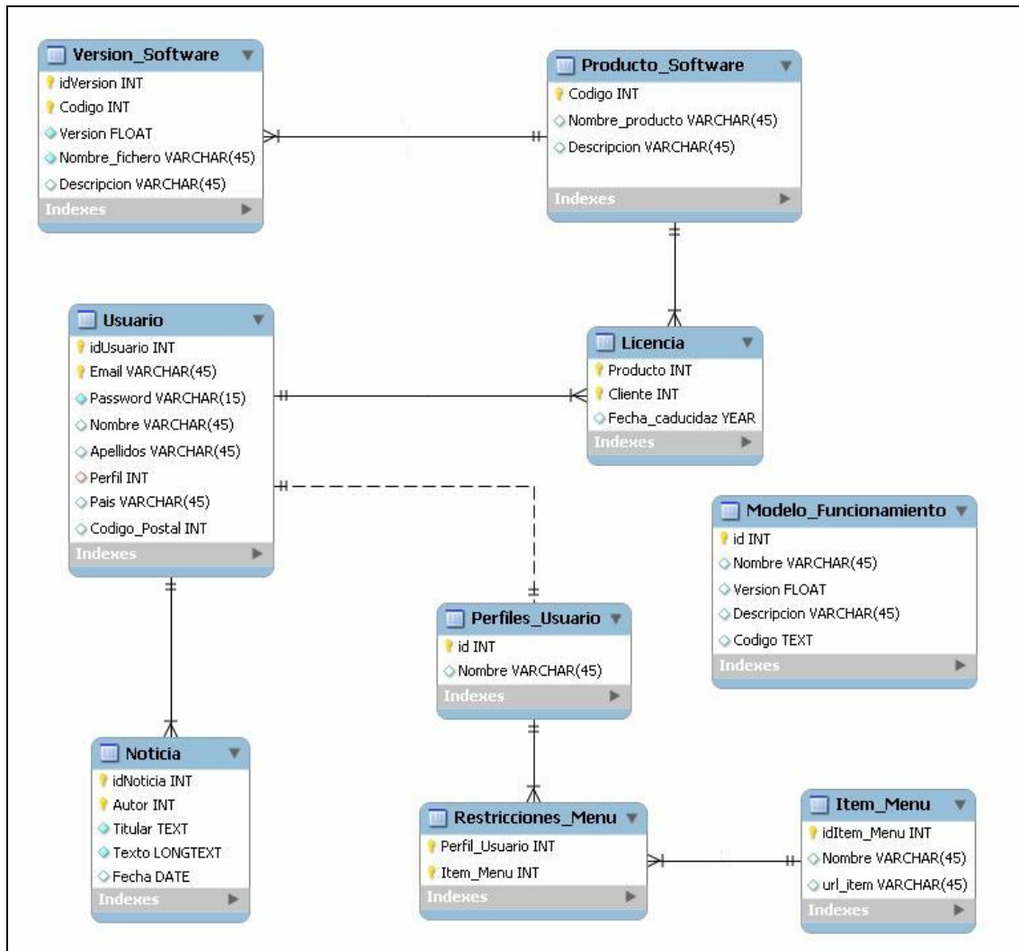
Figura 4.02: Estructura de la BBDD.
