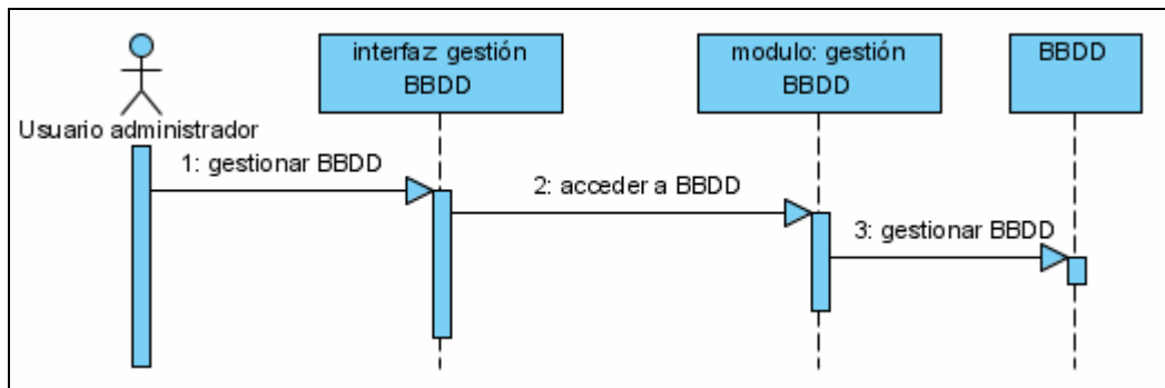
Fig. 3.25: Gestión de la BBDD.
