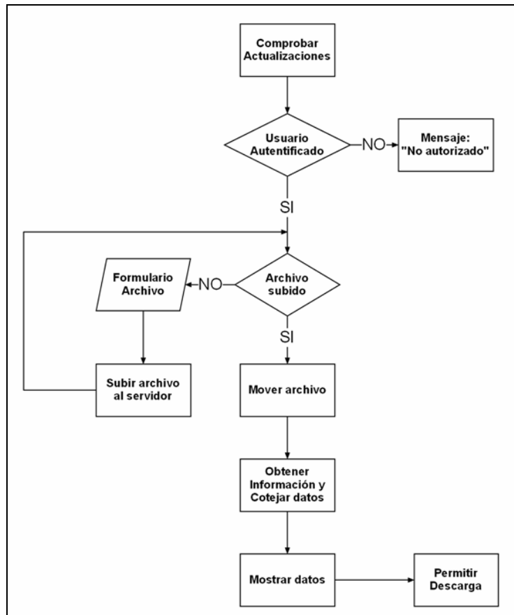
Fig. 5.6: Diagrama de flujo descargar actualizaciones.
