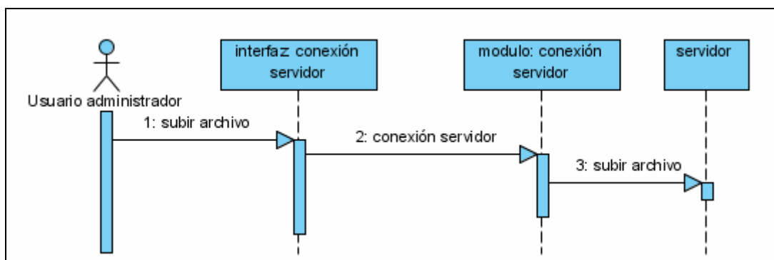
Fig. 3.24: Subir archivo al servidor.
