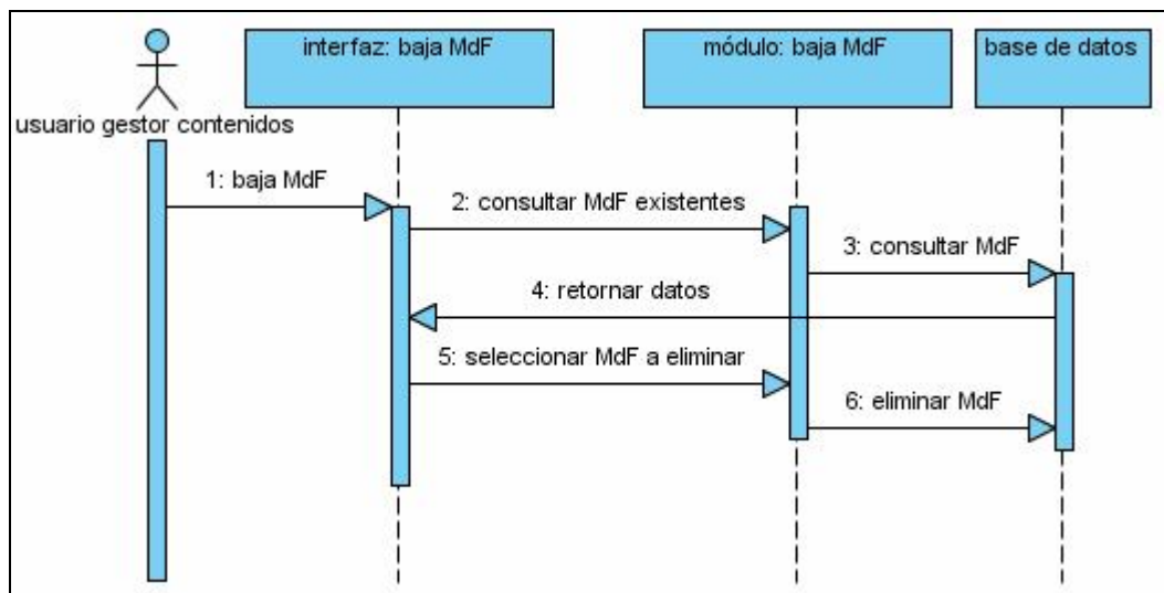
Fig. 17: Baja modelo de funcionamiento.
