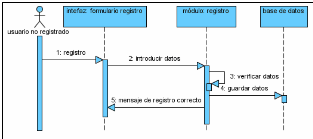
Fig.3.3: Registrarse
