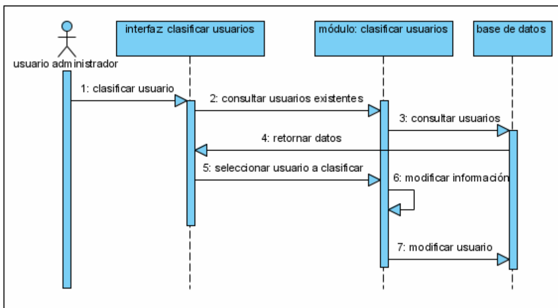
Fig. 3.22: Clasificar usuarios.
