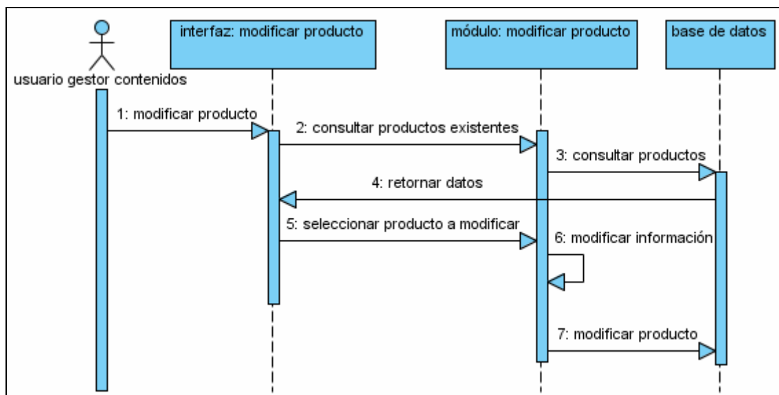
Fig. 3.15: Modificar producto.
