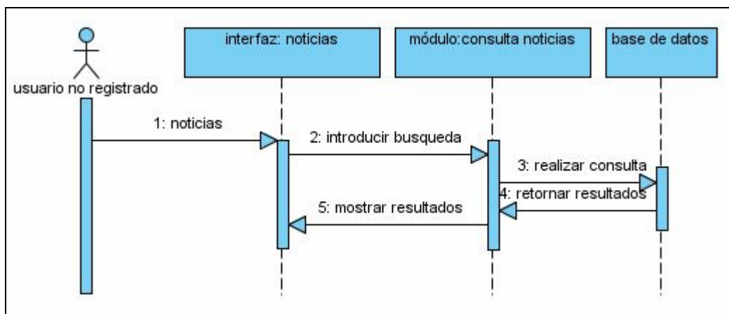
Fig.3.2: Consultar Noticias.
