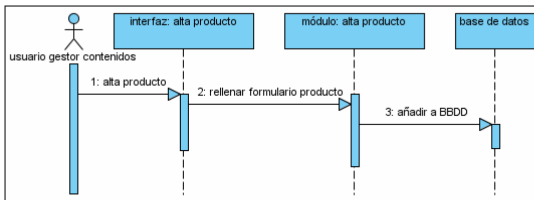
Fig. 3.13: Alta producto.
