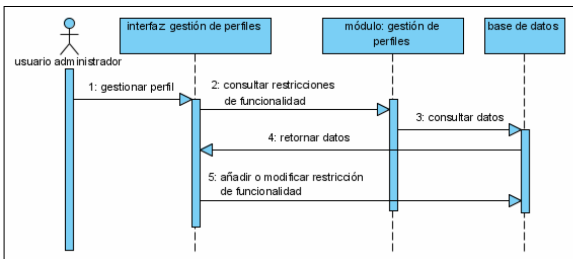
Fig. 3.23: Gestión de perfiles.
