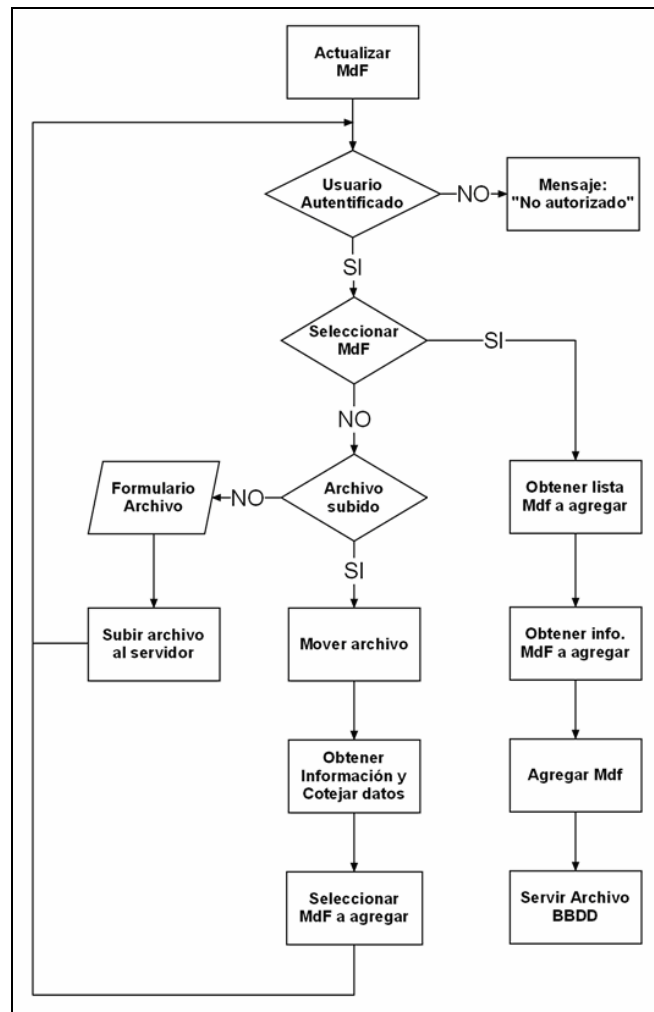
Fig. 6: Diagrama de flujo Actualizar lista MdF
