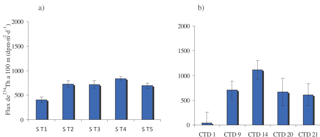
Fig. 13a Flux de 234 Th (dpm / m 2 dia) a 100 m de les cinc trapes de sediment (ST) de la primera campanya al març del 2009 i 13b, fluxos integrats de dèficit de Th-234 (dpm / m 2 dia) a 100 m derivats de la columna d'aigua per a cada CTD de la primera campanya.
