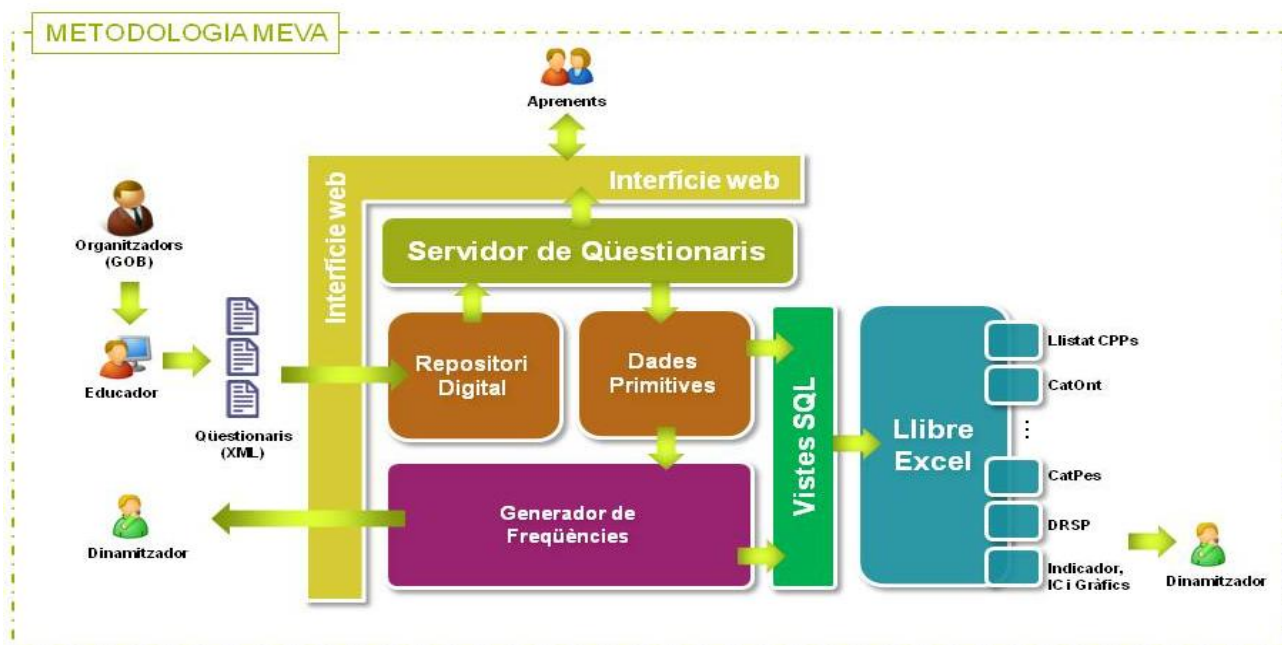
II-lustració 5: Solució conceptual de MEVA-Tool
