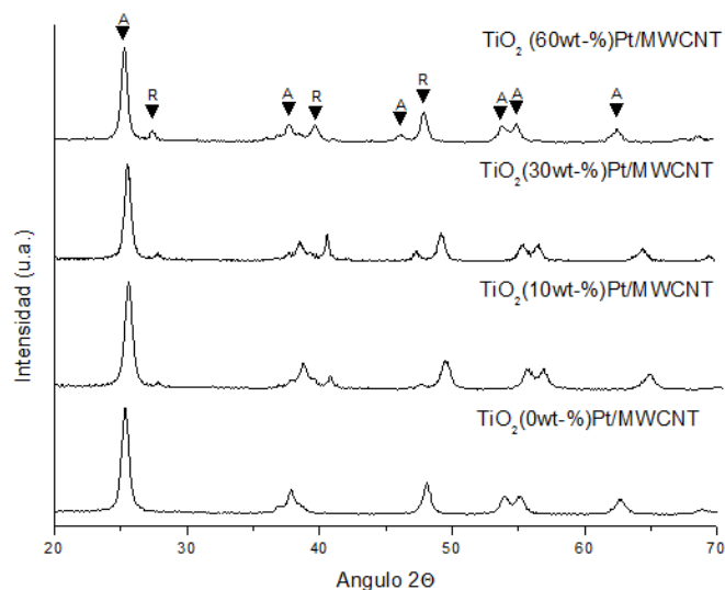
Fig. 4 Patrones de difracción de rayos X del \text{TiO}_2 puro y formando composites con MWCNT/Pt al 10, 20, 30 y 60%
