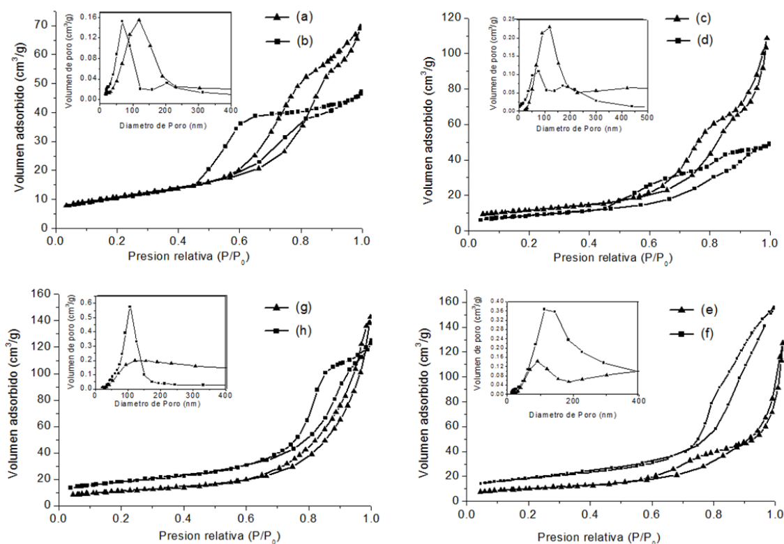
Fig. 6. Isothermas de adsorción-desorción de N_2 y curvas de distribución de tamaño de poro. (a) TiO_2/(5wt.\%)MWCNT/Pt(20nm) , (b) TiO_2/(5wt.\%) MWCNT/Pt (60nm) , (c) TiO_2/(10wt.\%)MWCNT/Pt(20nm) , (d) TiO_2/(10wt.\%)MWCNT/Pt (60nm) , (e) TiO_2/(30wt.\%)MWCNT/Pt(20nm) , (f) TiO_2/(30wt.\%)MWCNT/Pt(60nm) , (g) TiO_2/(60wt.\%)MWCNT/Pt(20nm) , (h) TiO_2/(60wt.\%)MWCNT/Pt(60nm) .
