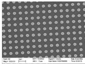
Fig. 1: Imatge de les estructures circulars, fabricades mitjançant litografia per feix d'electrons, obtinguda per microscòpia electrònica.
