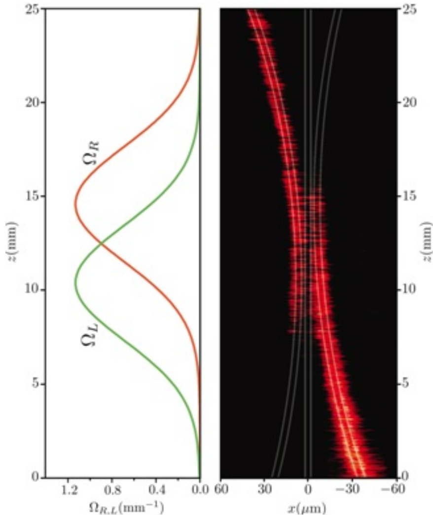
A l'esquerra, seqüència dels acoblaments entre les guies mesurats experimentalment en de la direcció de propagació de la llum. A la dreta, vista superior d'un dels dispositius fabricats en el qual es pot observar la transferència completa de llum entre les guies laterals del sistema.
